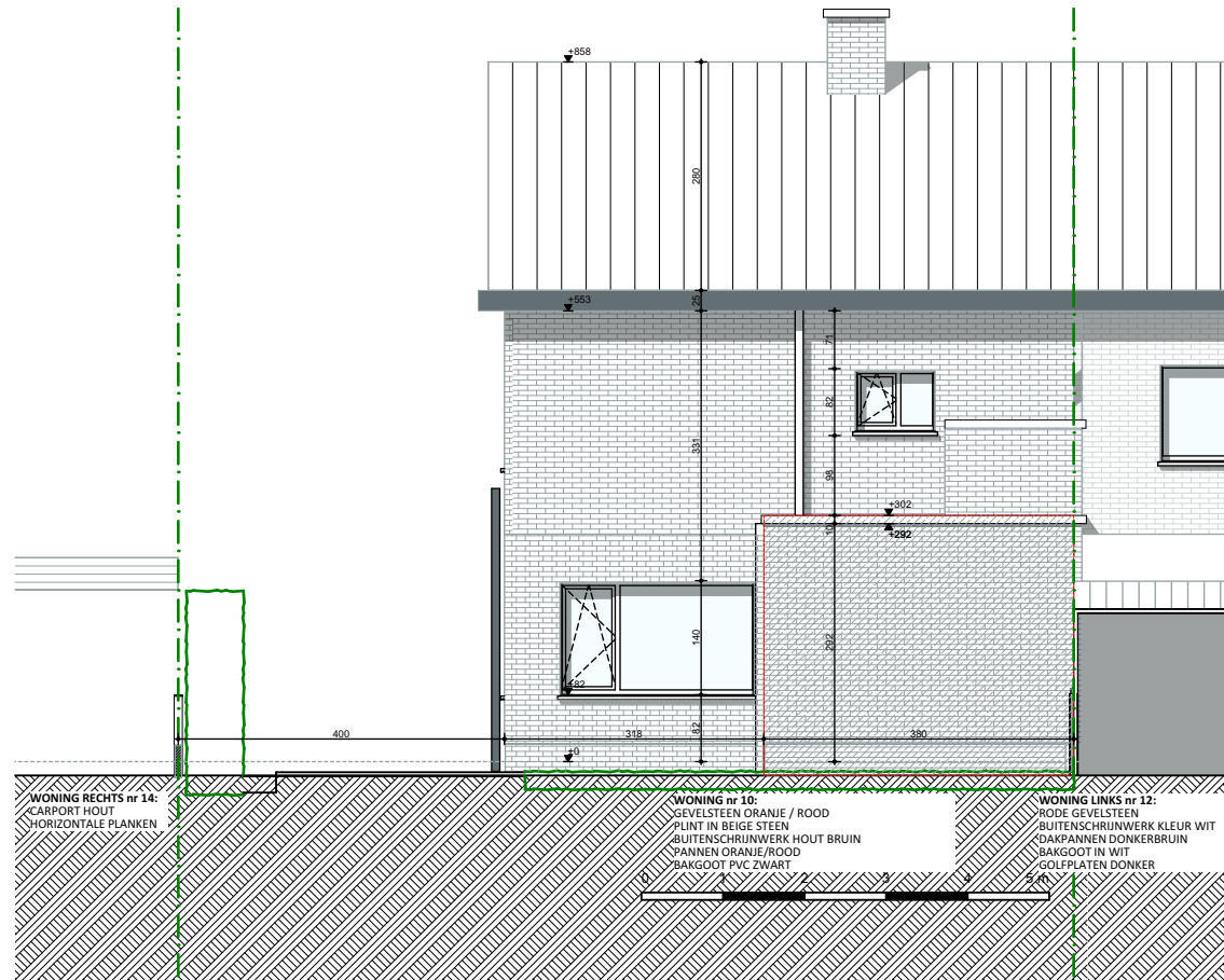
ACHTERGEVEL - Bestaande toestand
