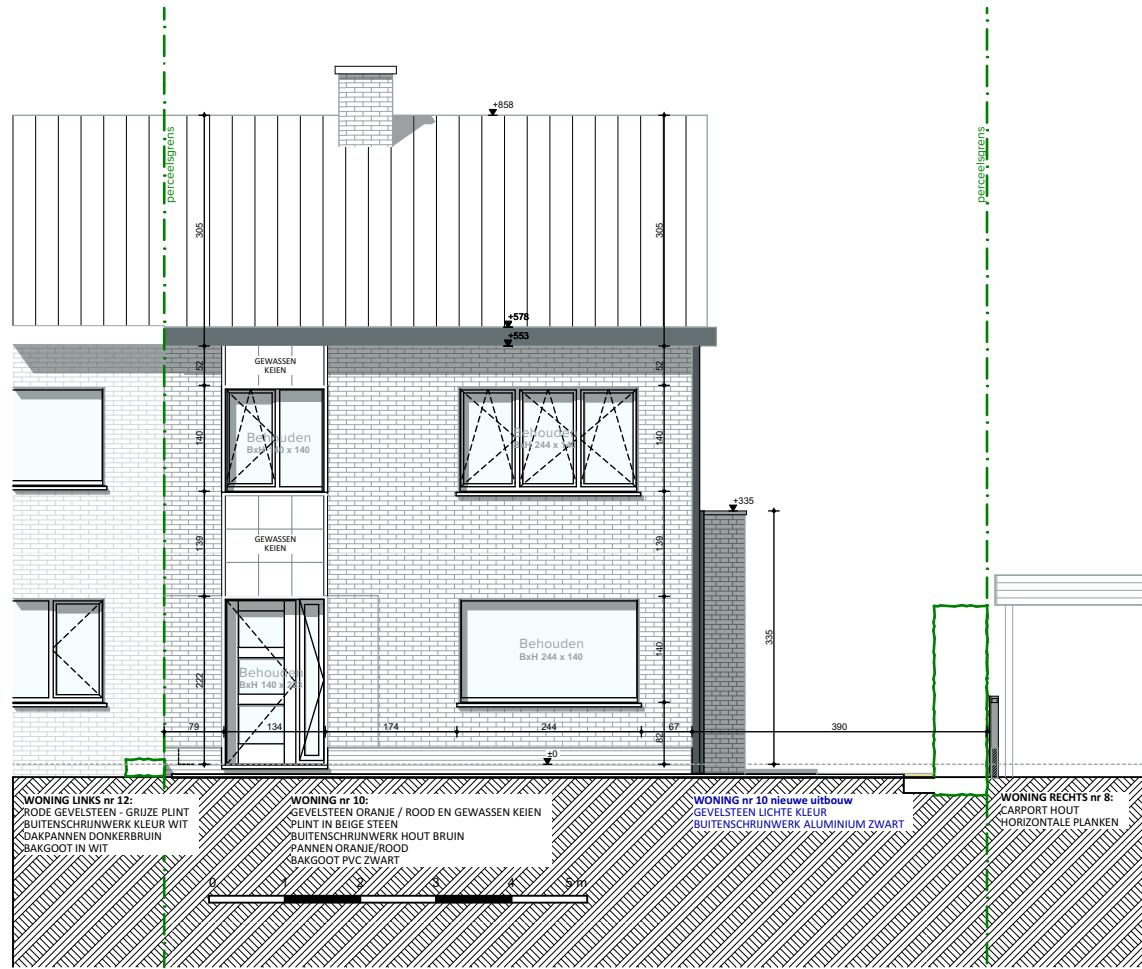
VOORGEVEL - Nieuwe toestand
