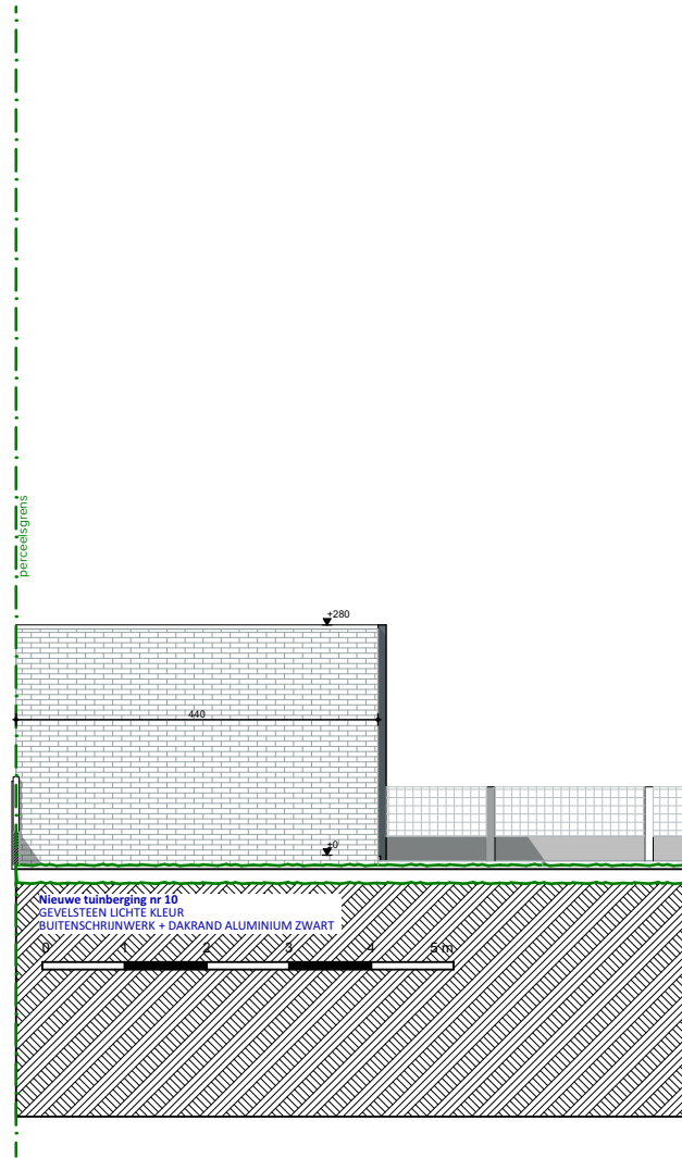
LINKERGEVEL TUINBERGING 1:100
