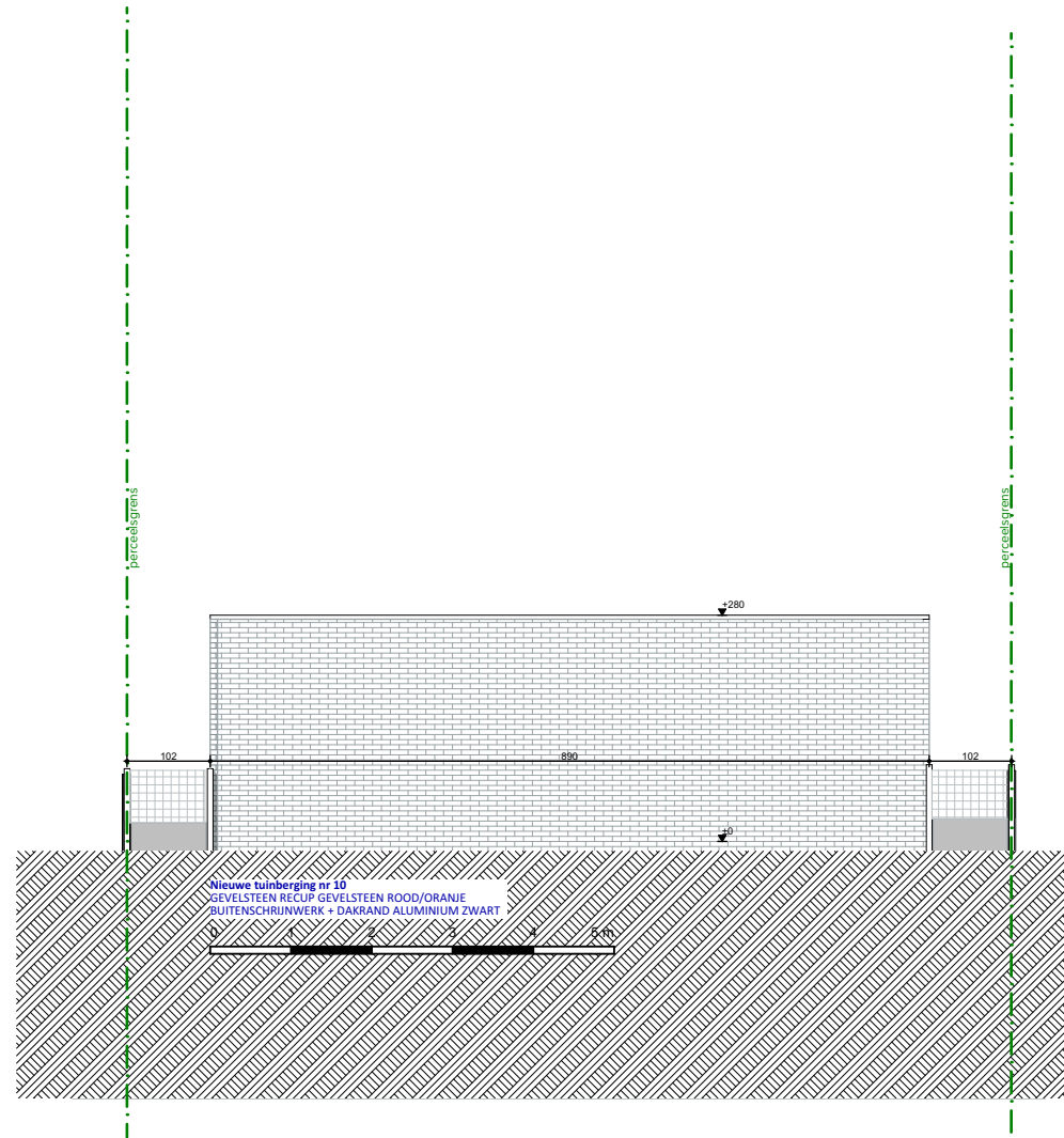
ACHTERGEVEL TUINBERGING
