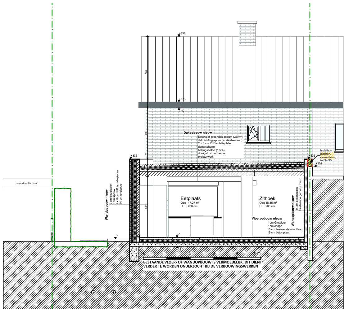
DOORSNEDE S3 - Nieuwe toestand
