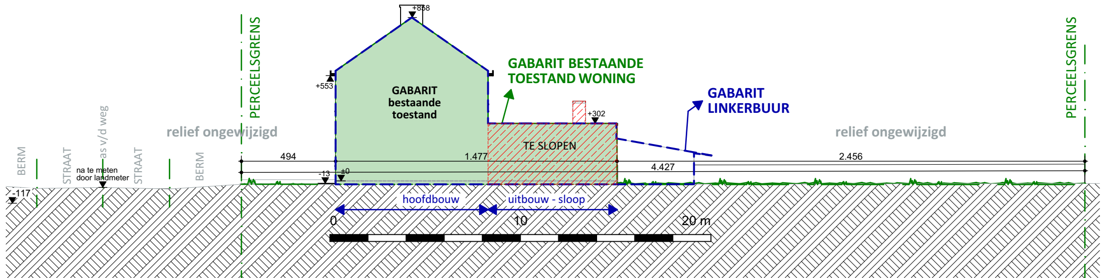
TERREINPROFIEL - Bestaande toestand
