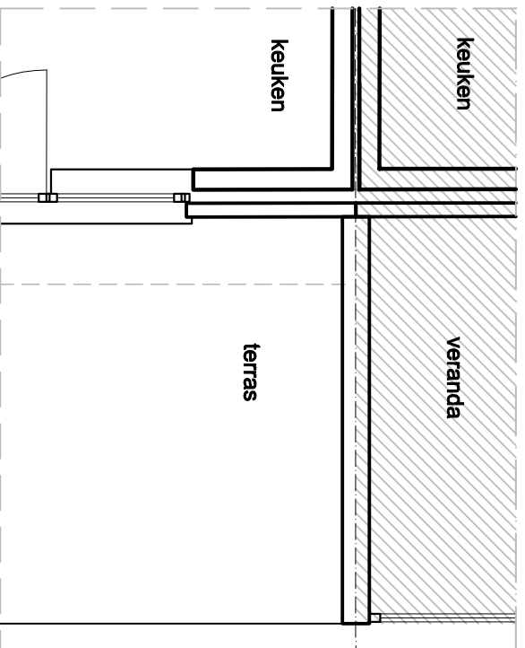
grondplan
