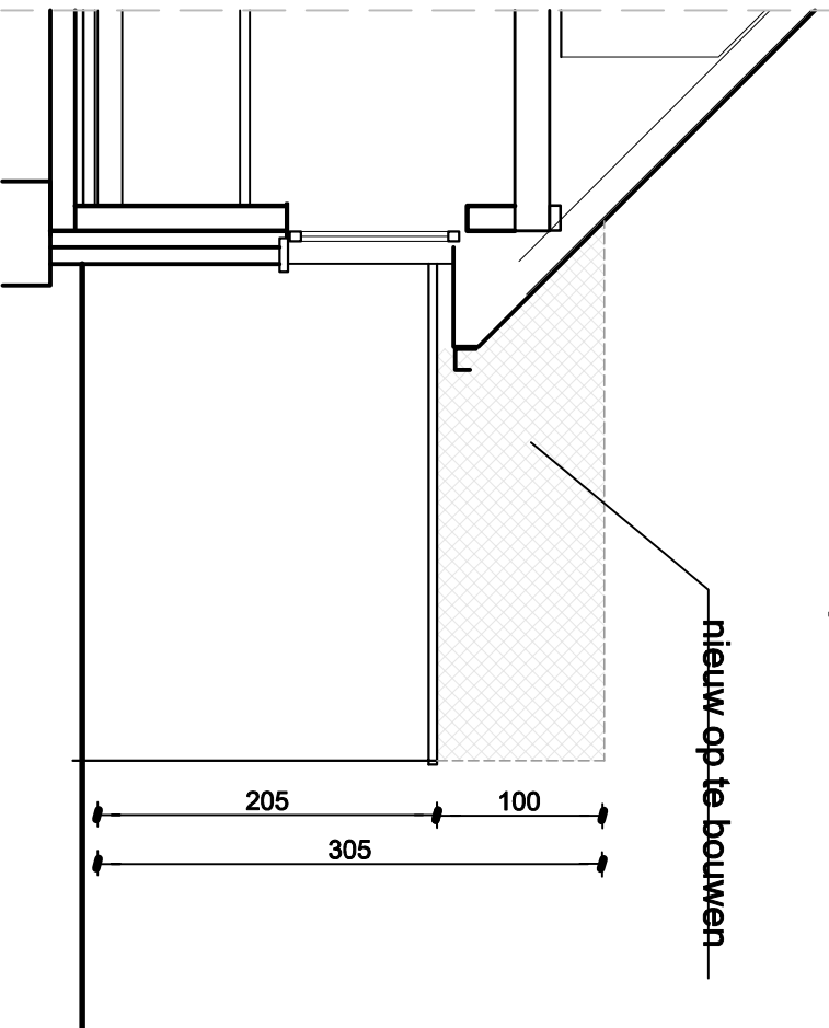
doorsnede zijaanzicht
