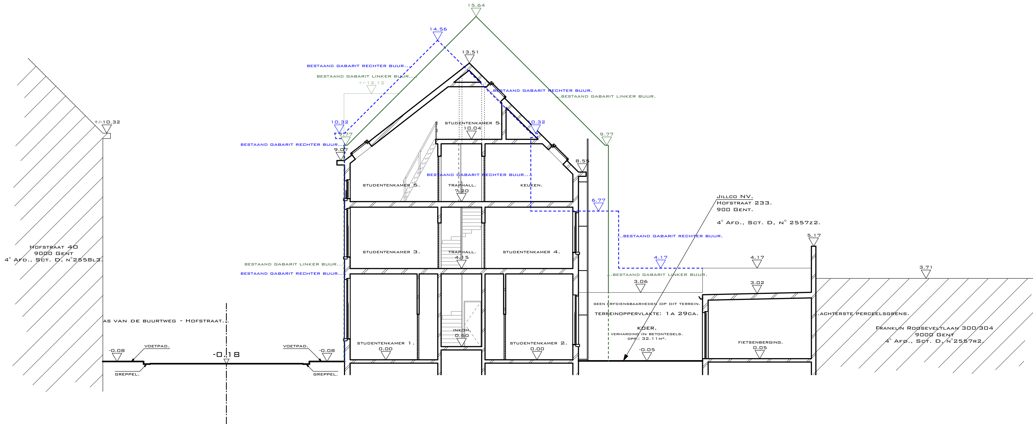
TERREINPROFIEL A - BESTAANDE TOESTAND - SCHAAL: 1/100.
