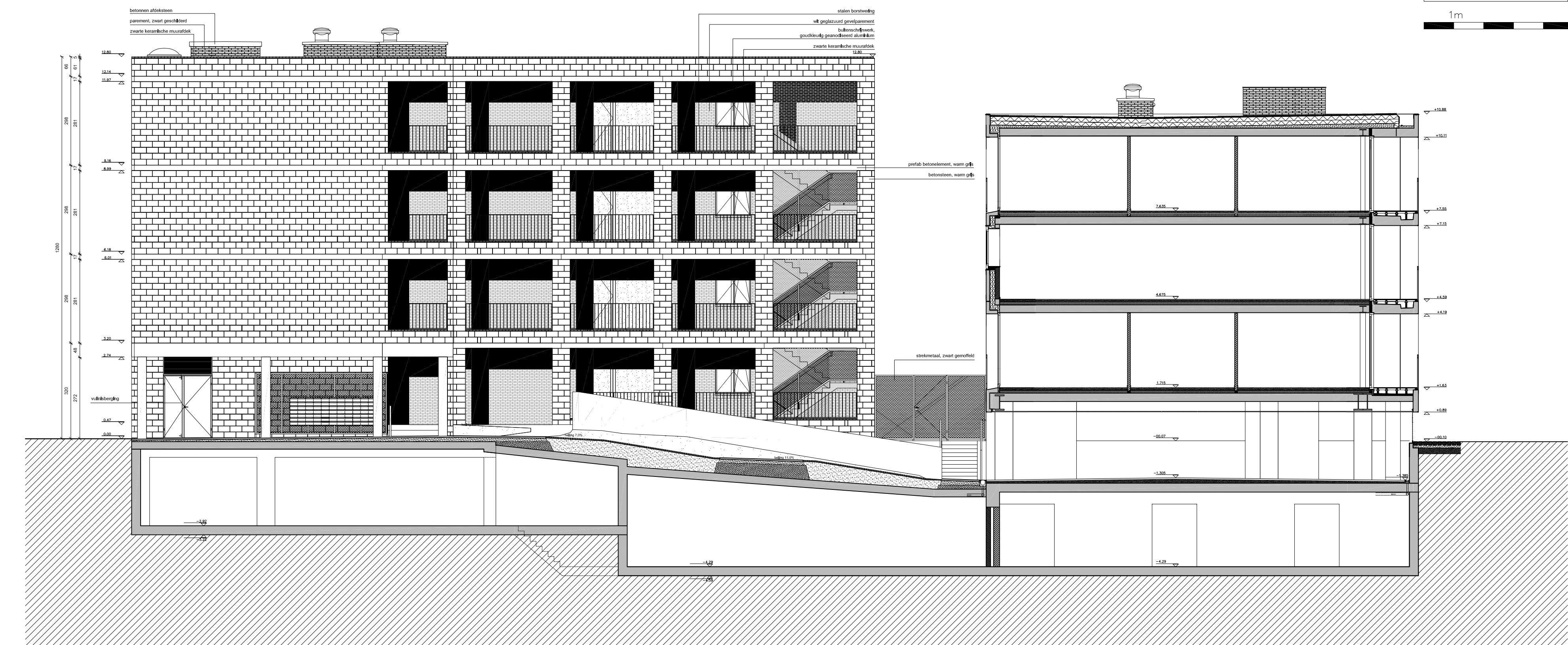
2. BLOK B gevel noord - BLOK A snede
