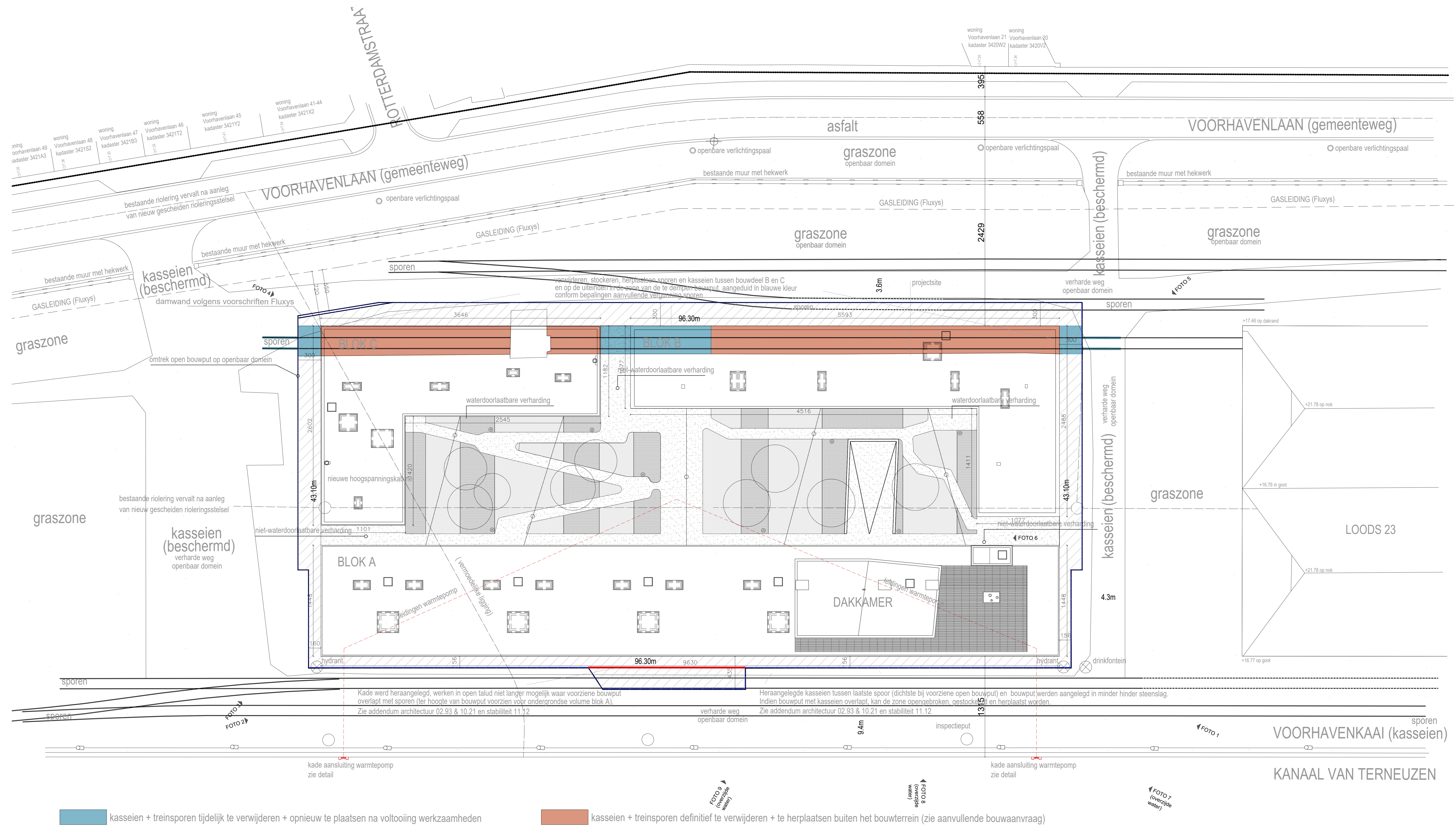
Inplantingsplan, schaal 1/200
