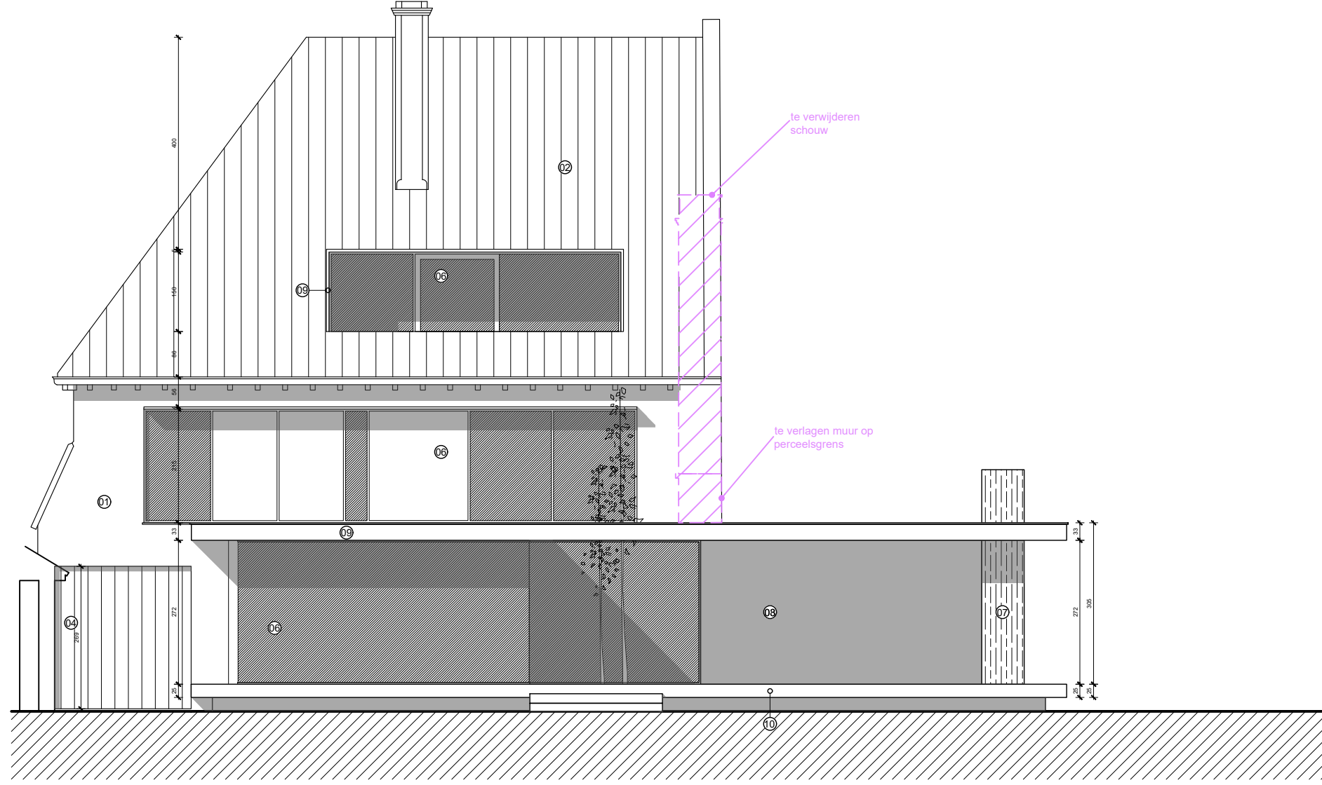
ZICHT ACHTERGEVEL NIEUWE TOESTAND
