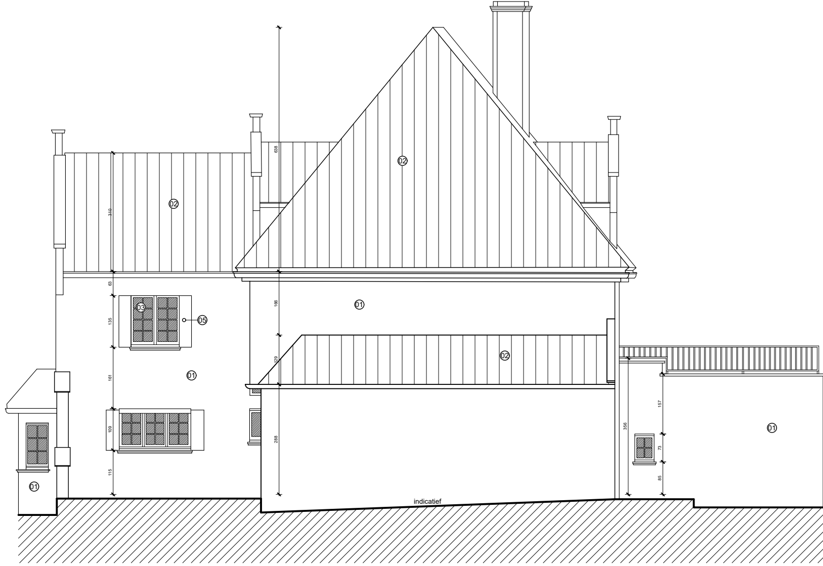
ZICHT RECHTERGEVEL BESTAANDE TOESTAND
