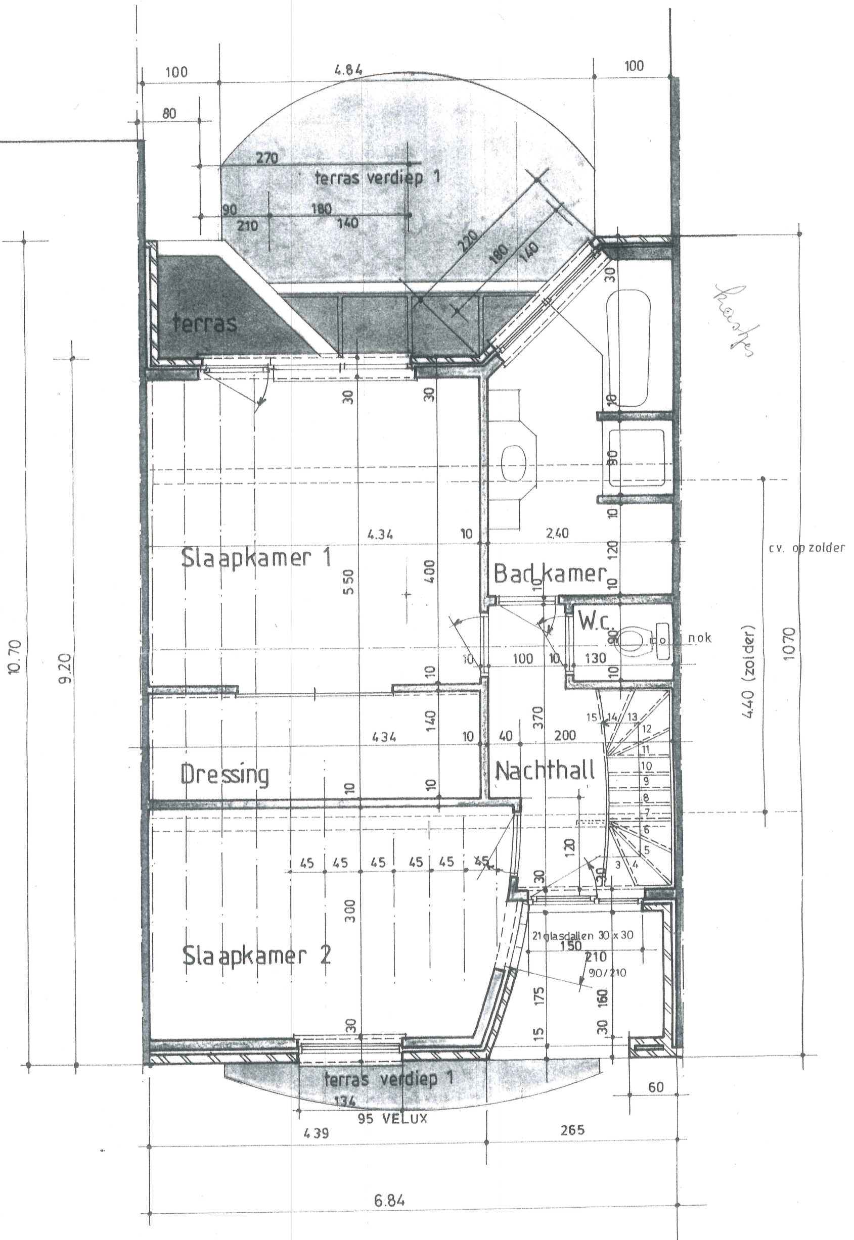
Plan verdiep 2
