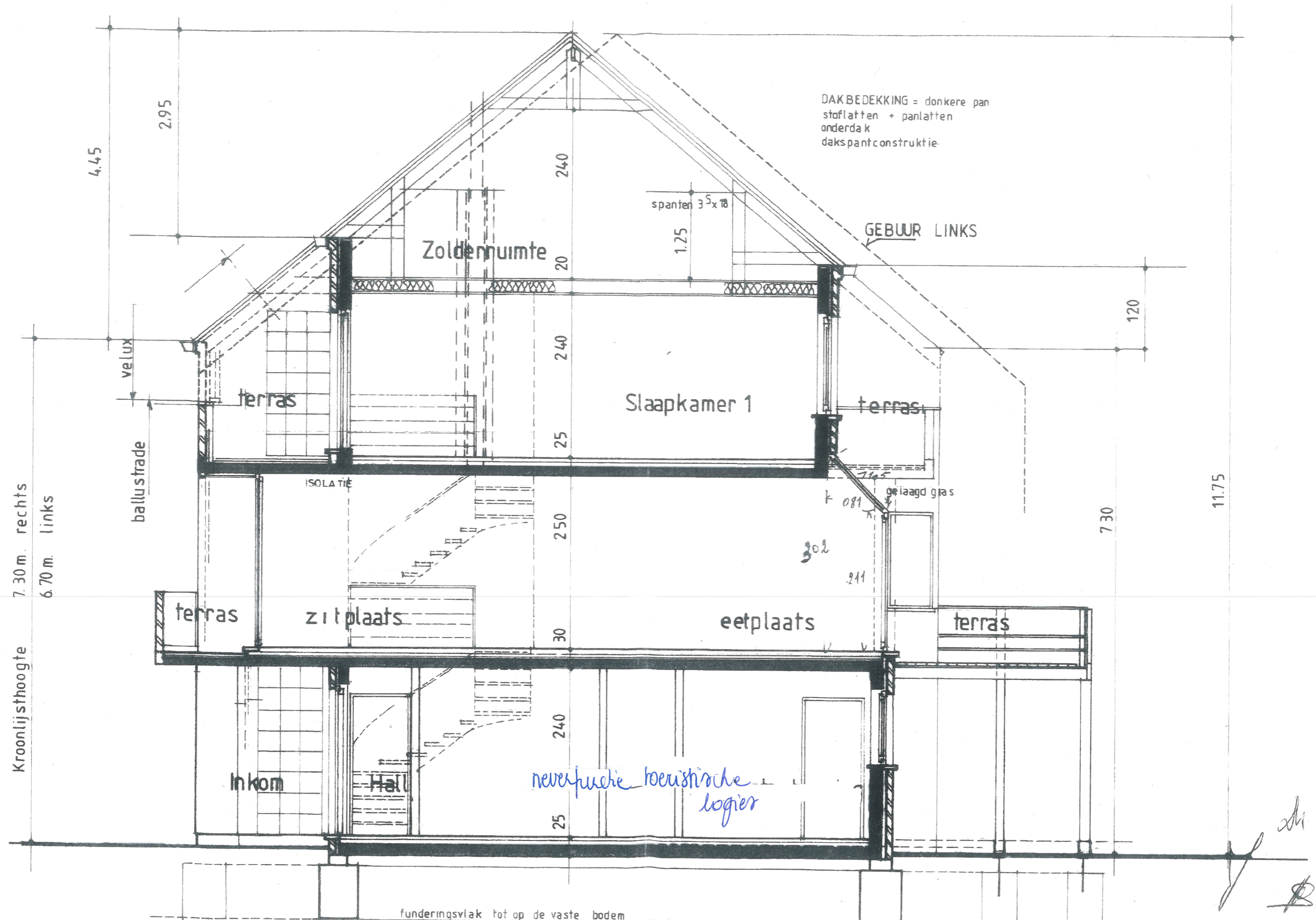
Doorsnede 2-2
