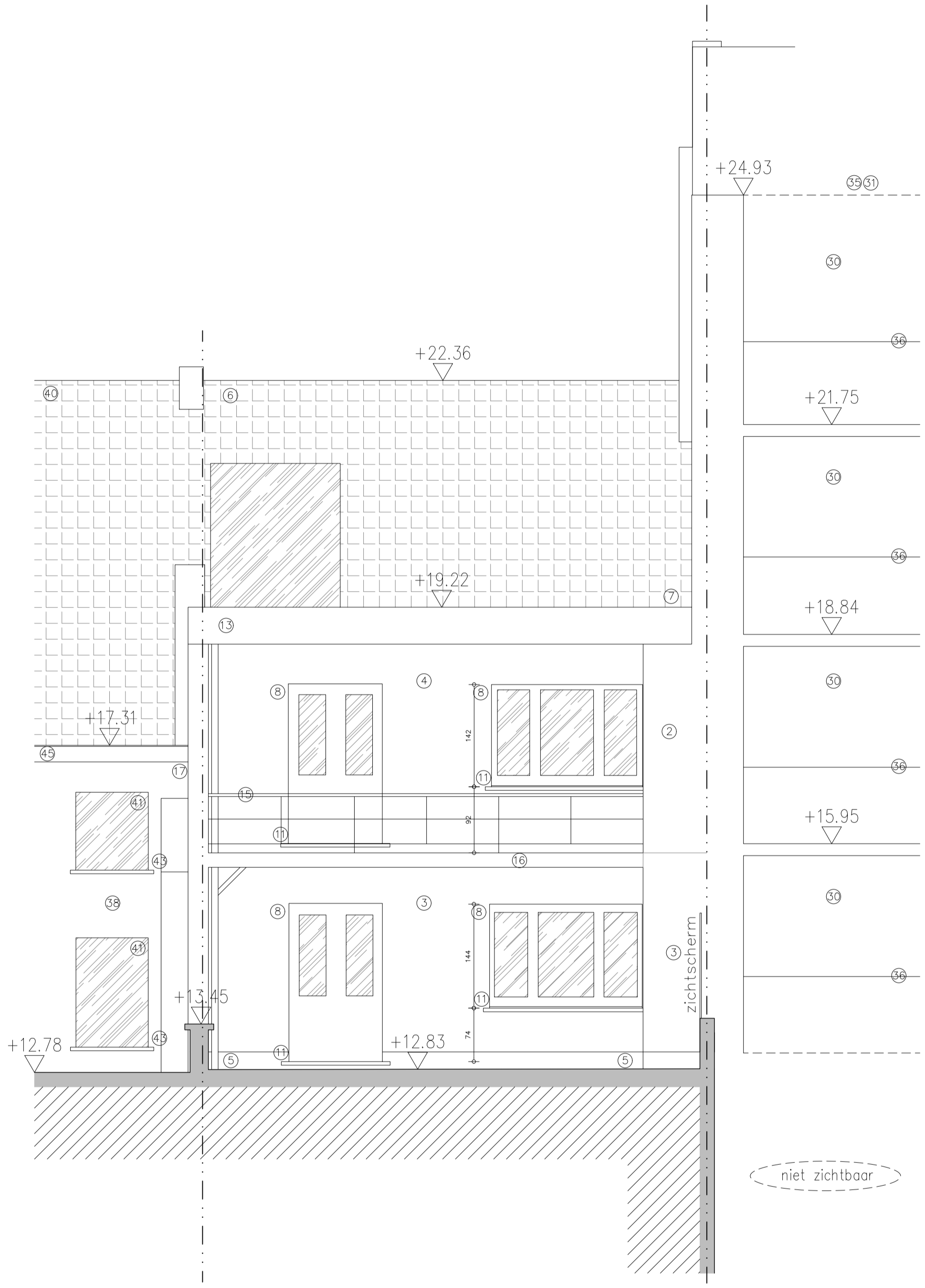
ACHTERGEVEL bestaand schaal 1/200
