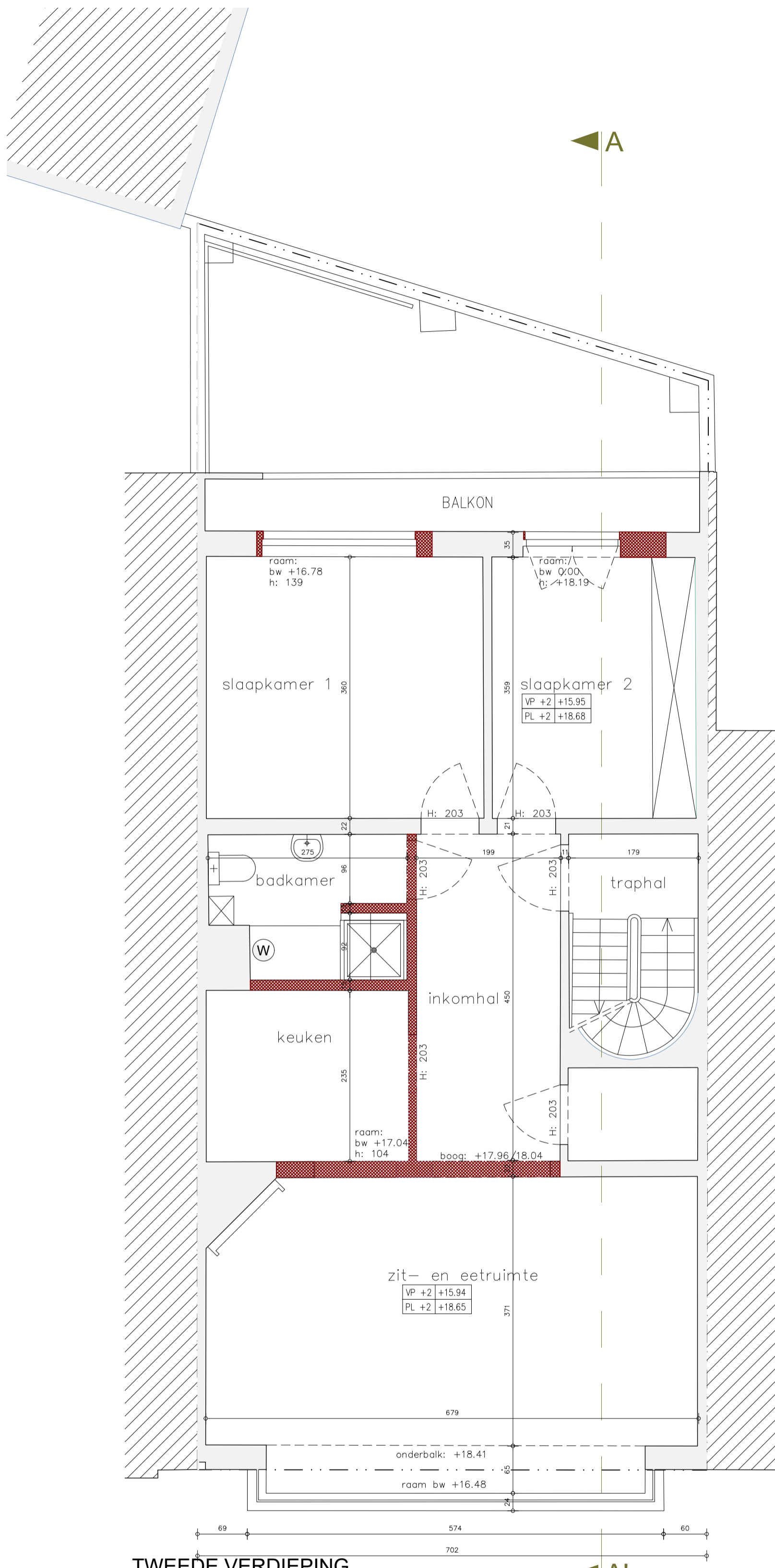
TWEDE VERDIEPING bestaand schaal 1/50
