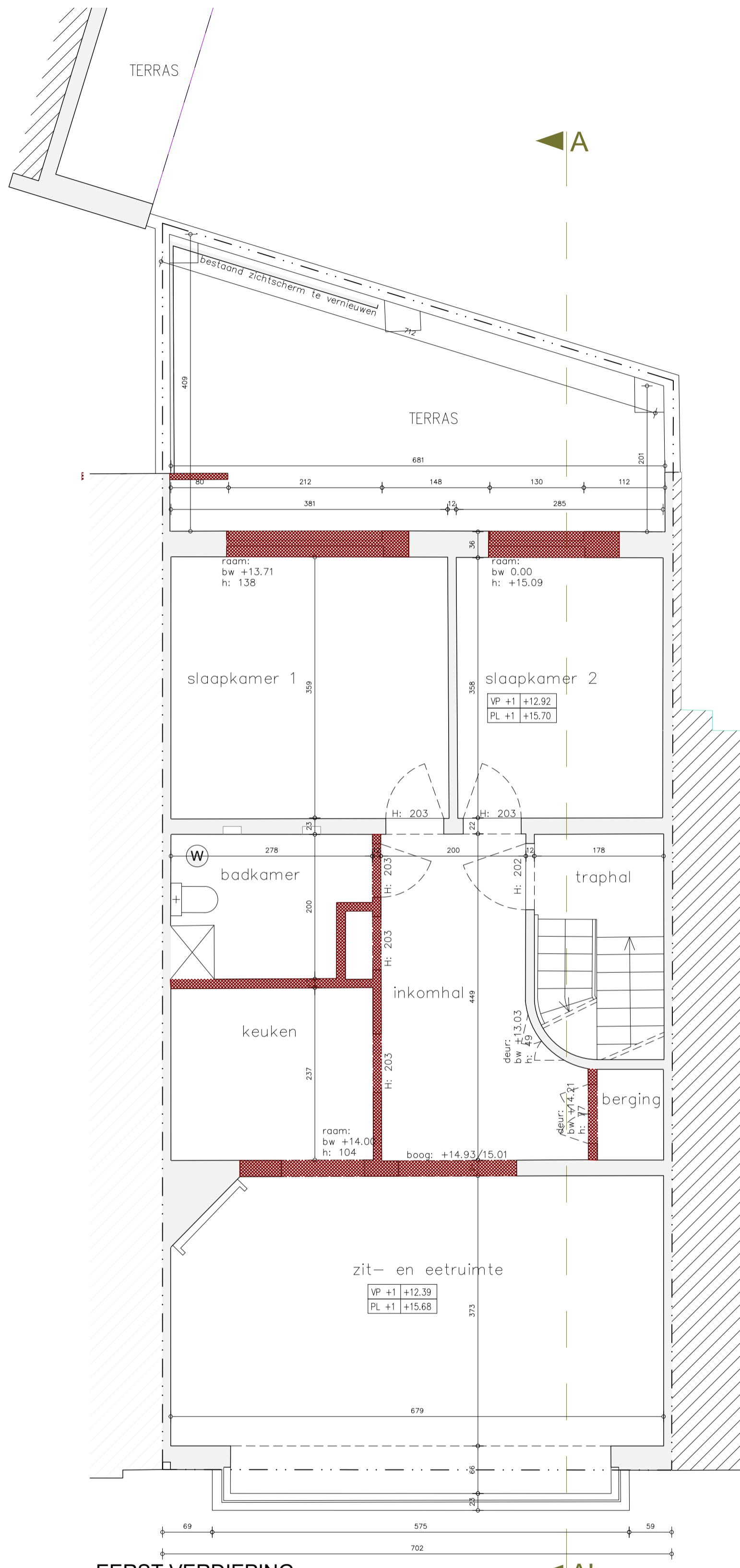
EERST VERDIEPING bestaand schaal 1/50
