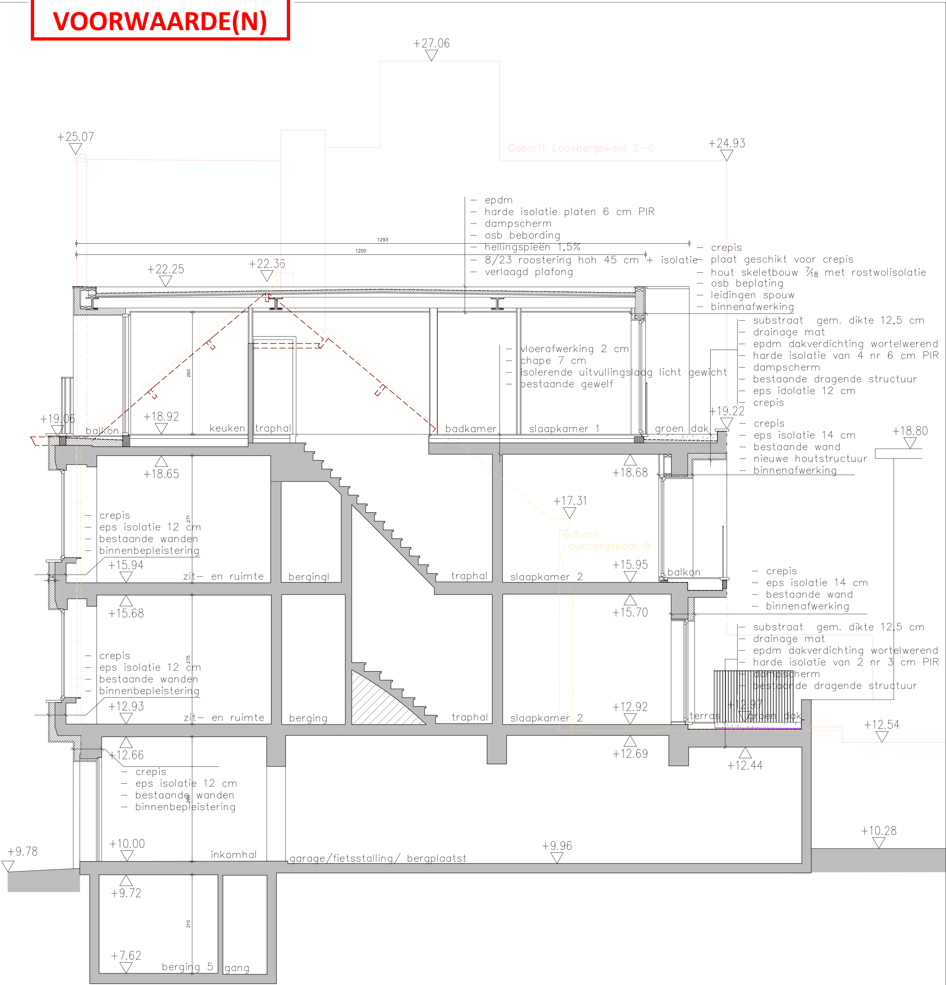
DOORSNEDE AA' nieuw schaal 1/50
