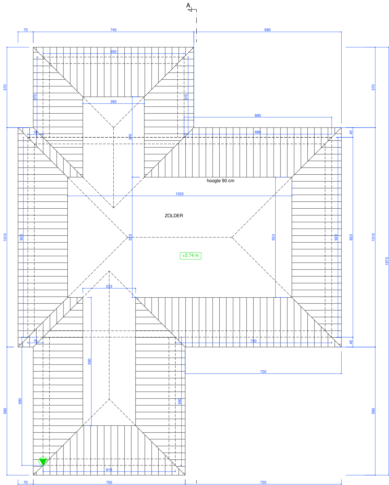
ZOLDERPLAN bestaande toestand
