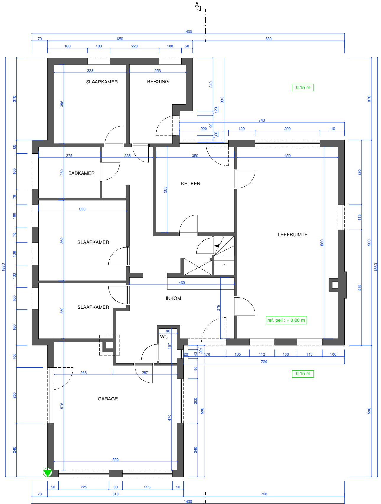
GRONDPLAN bestaande toestand
