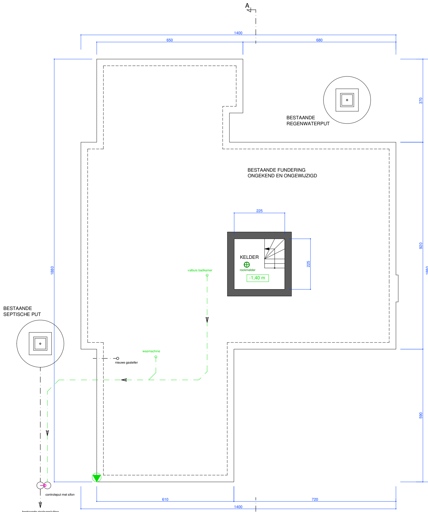
KELDER EN FUNDERINGSPLAN nieuwe toestand
