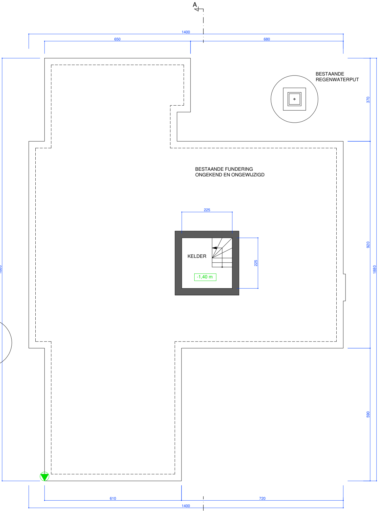
KELDER EN FUNDERINGSPAN bestaande toestand
