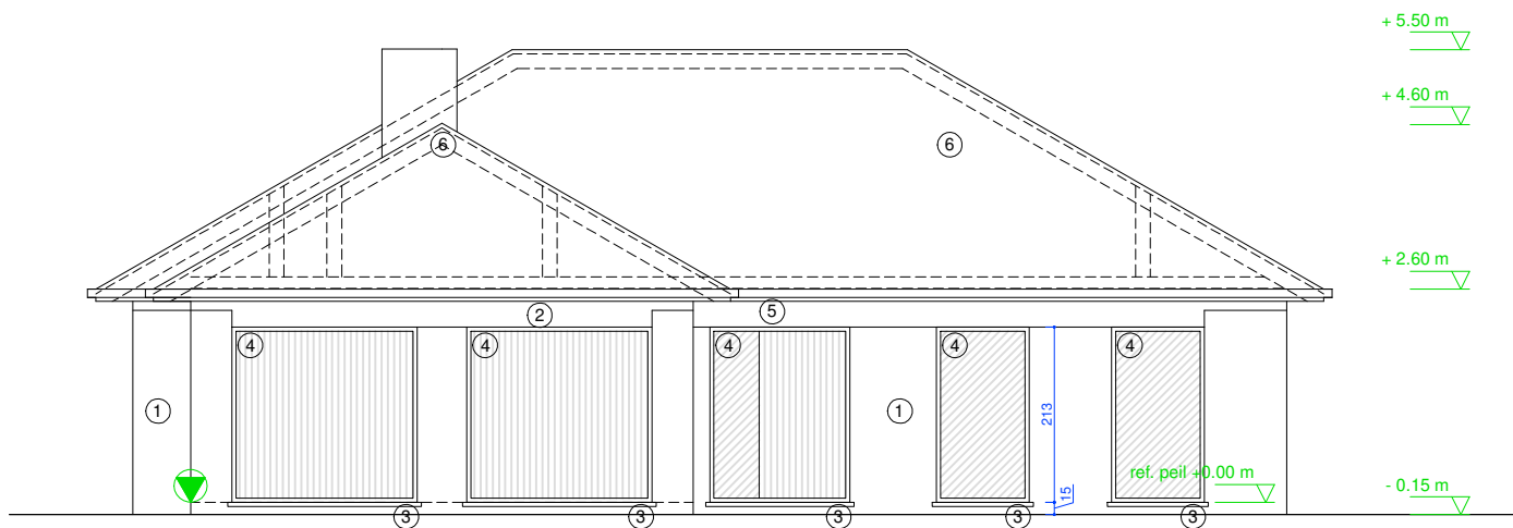
VOORGEVEL bestaande toestand
