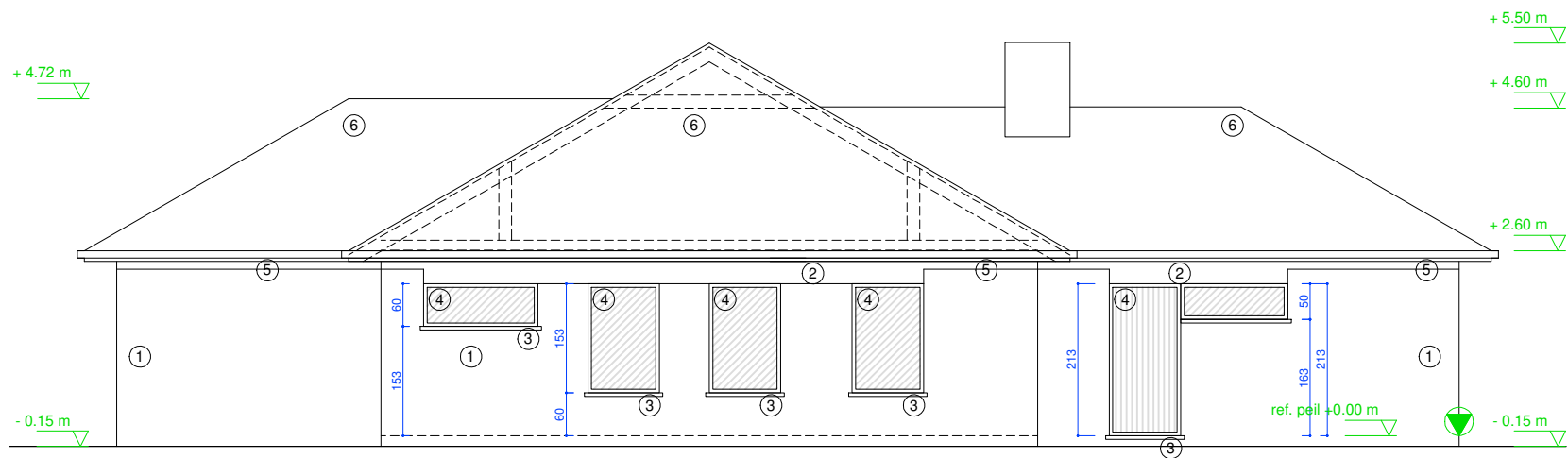
ZIJGEVEL LINKS bestaande toestand
