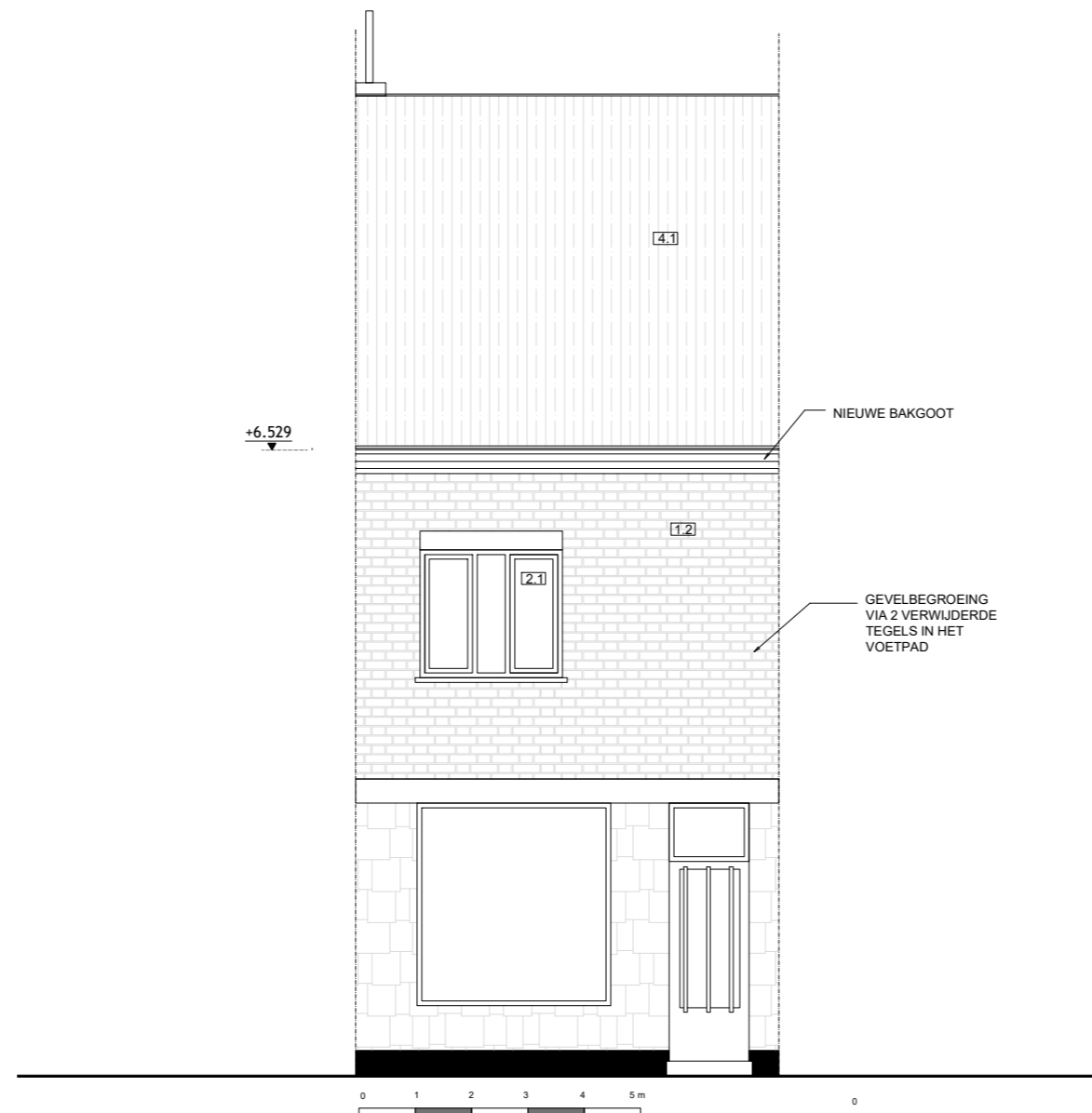
Voorgevel BT Maateenheid: Millimeter Schaal : 1:125
