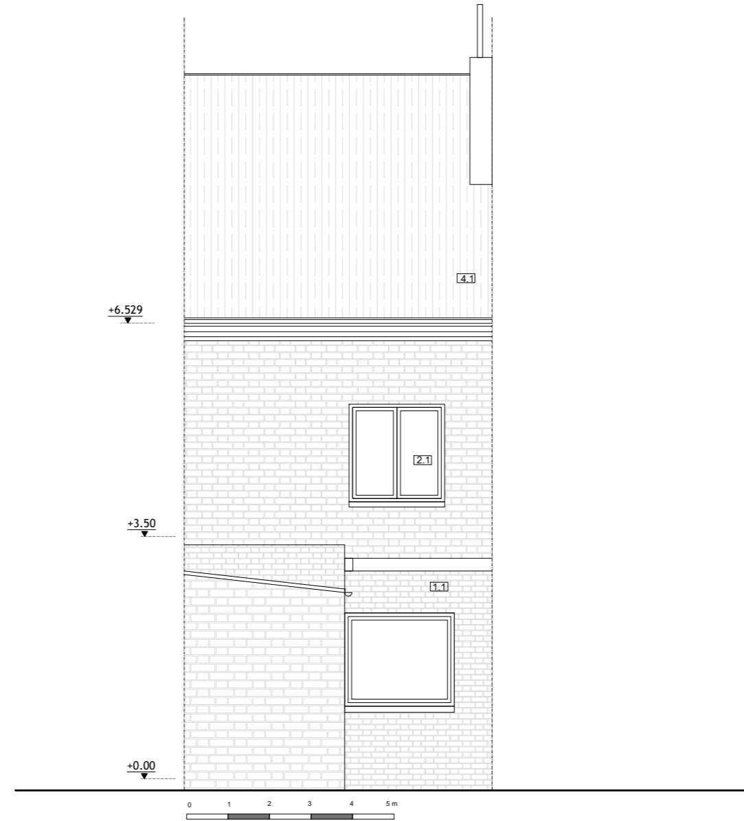
Achtergevel BT Maateenheid: Millimeter Schaal : 1:125
