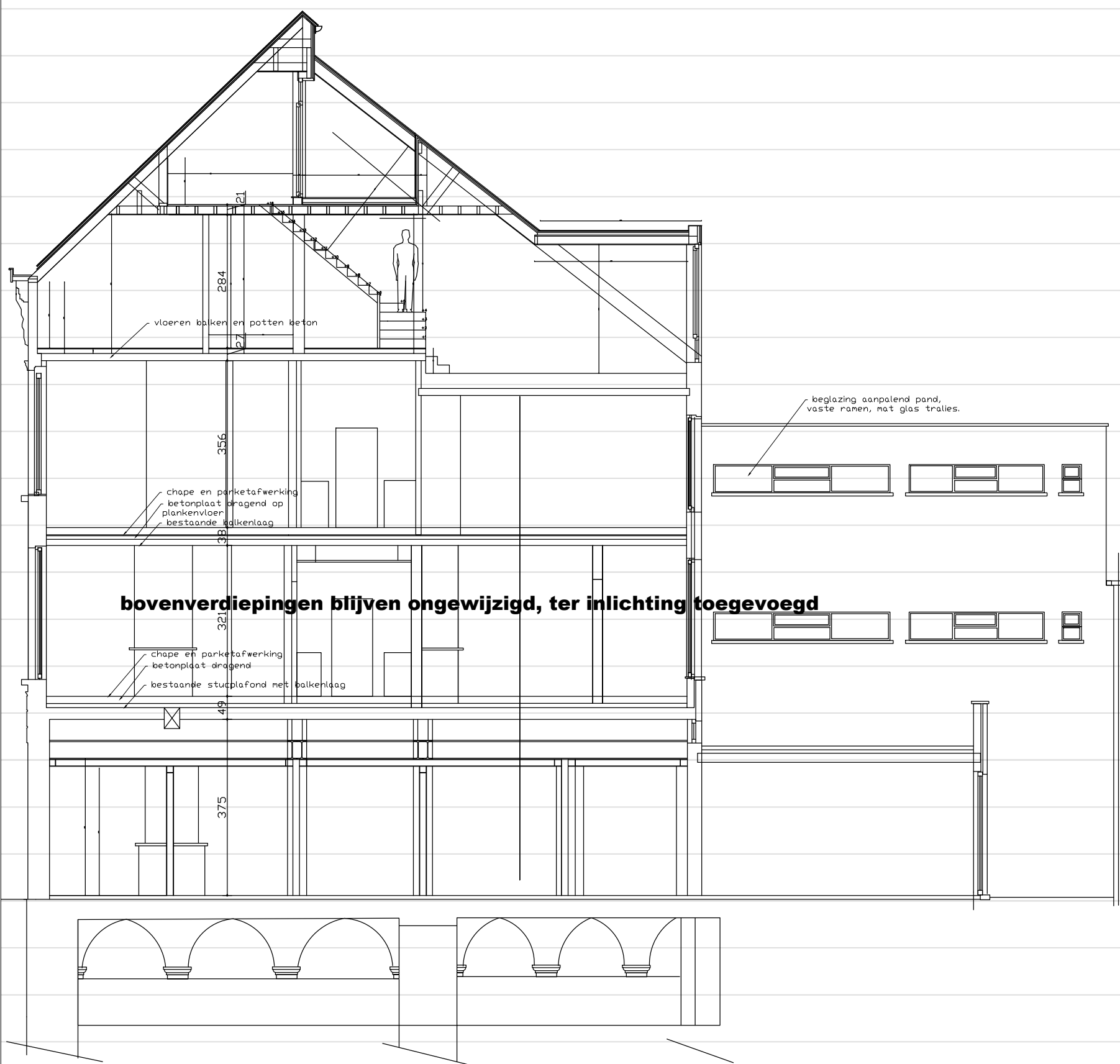
Doorsnede C - D
