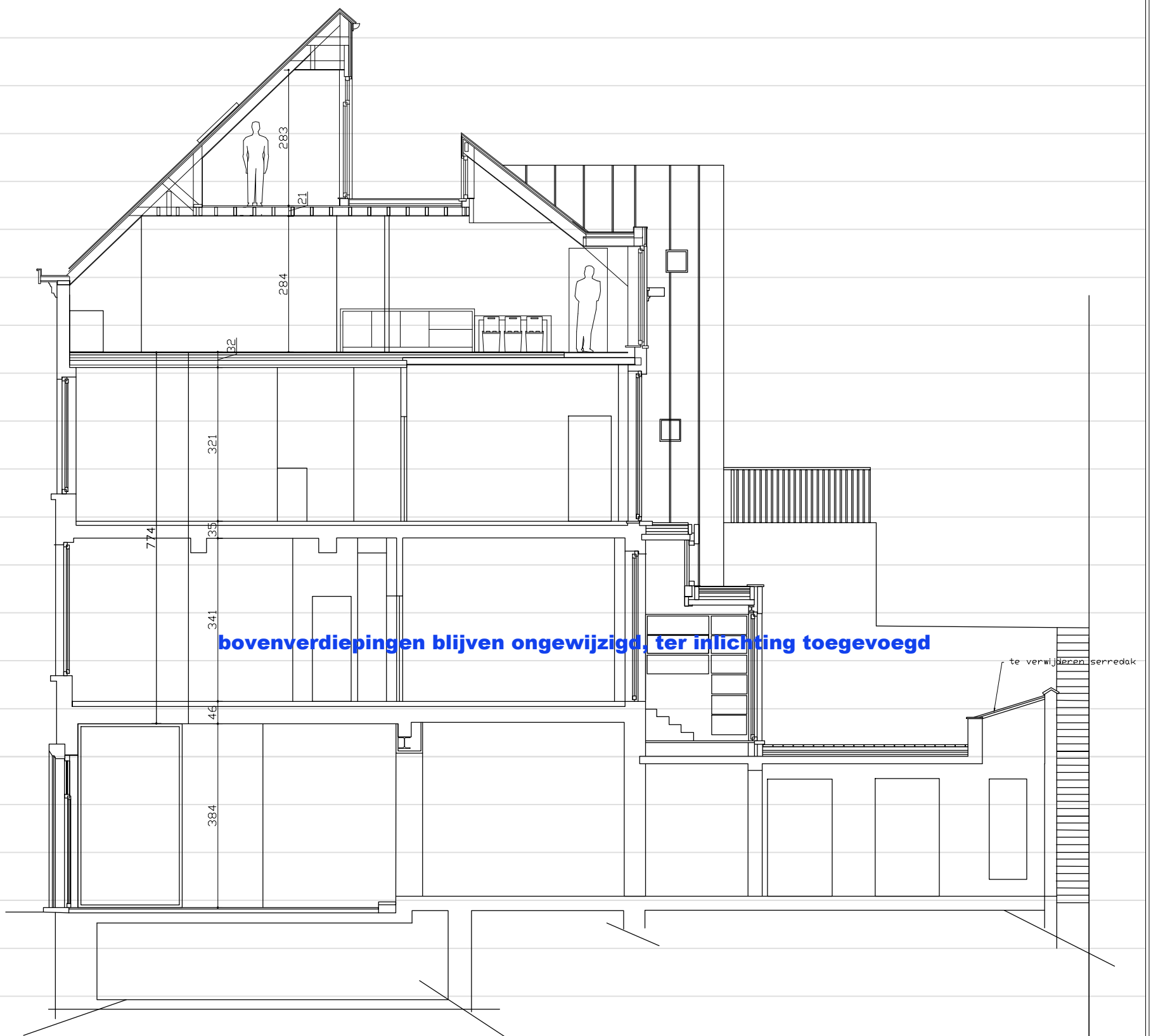
Doorsnede A - B
