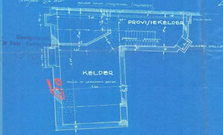
KELDERPLAN.
