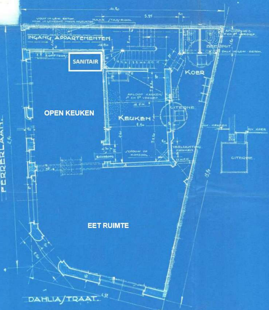
GELIJKVLOERPLAN.
