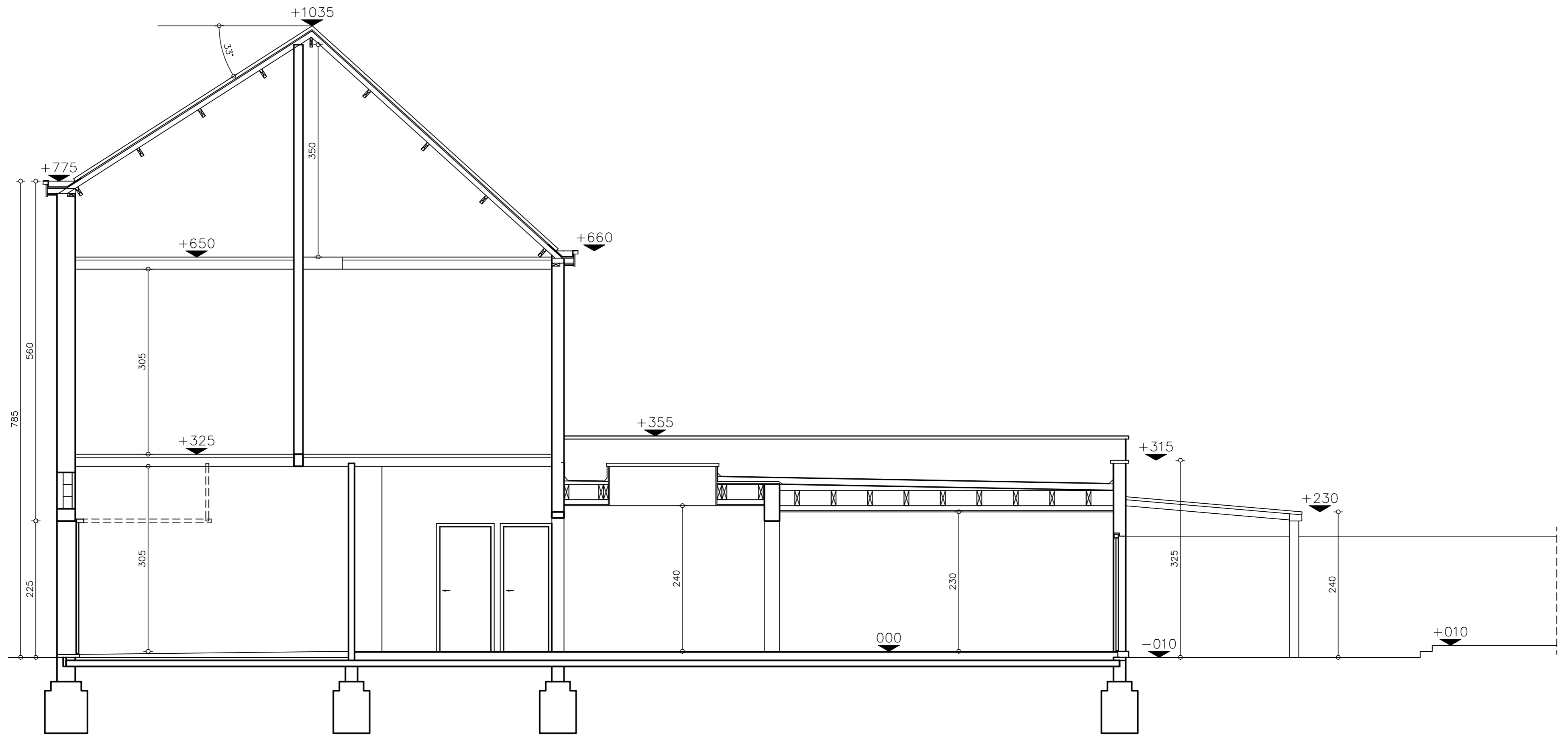
DOORSNEDE AA bestaande toestand SCHAAL 1/50
