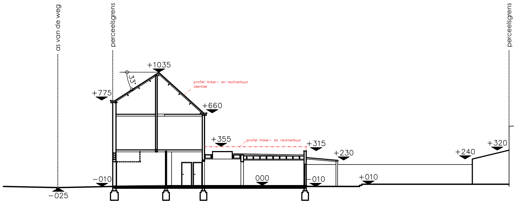
TERREINPROFIEL bestaende toestand SCHAAL 1/200
