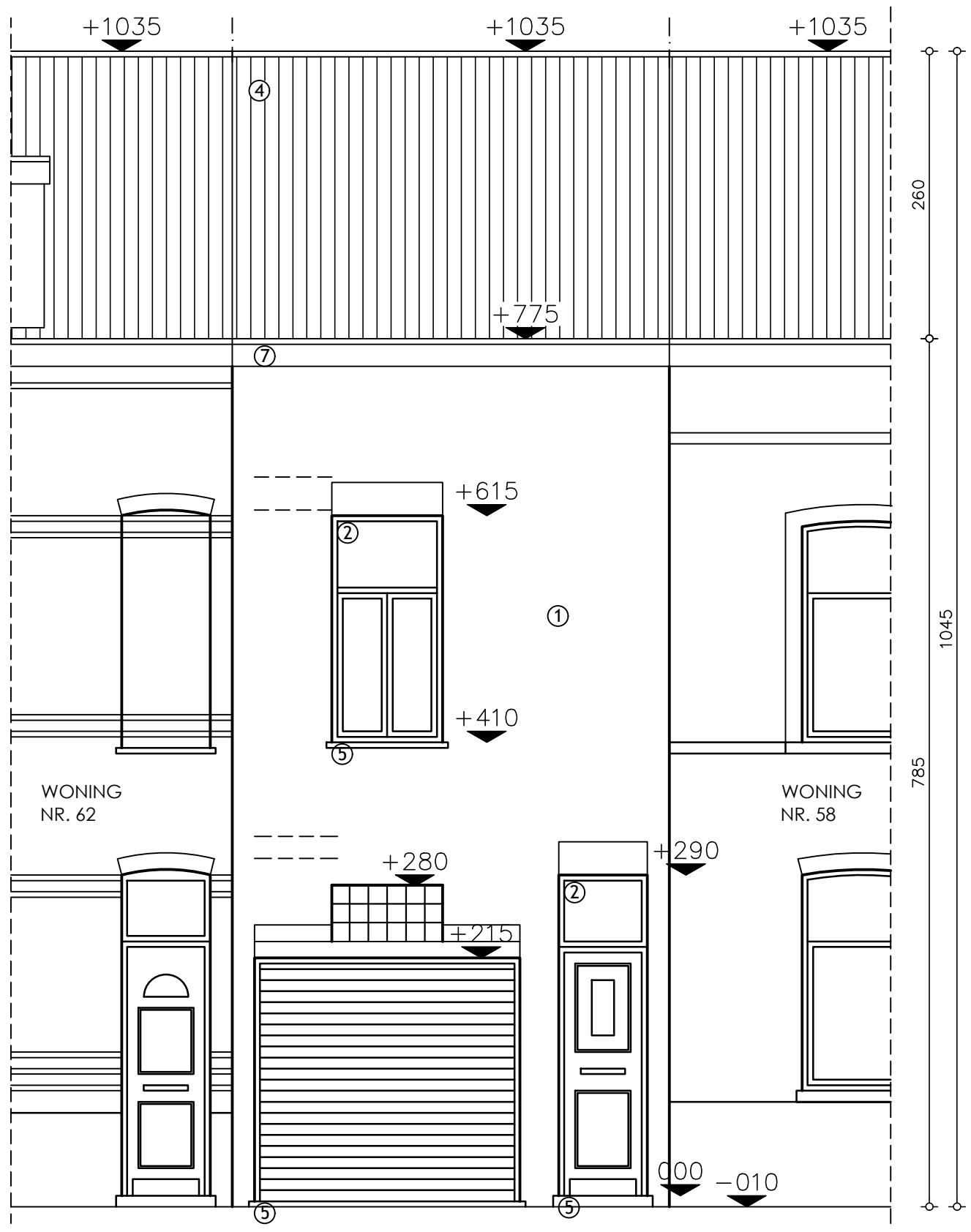
VOORGEVEL bestaande toestand SCHAAL 1/50
