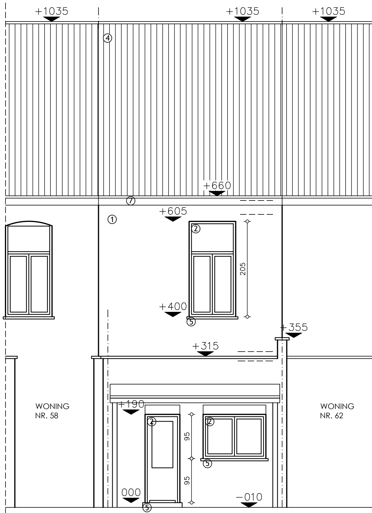
ACHTERGEVEL bestaande toestand SCHAAL 1/50
