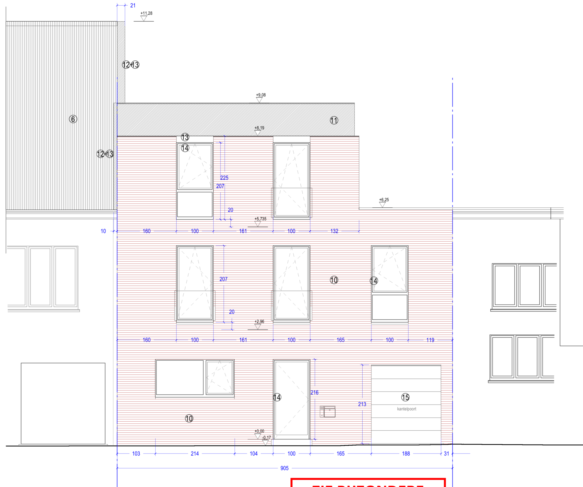
VOORGEVEL (straatzijde) - nieuwe toestand
