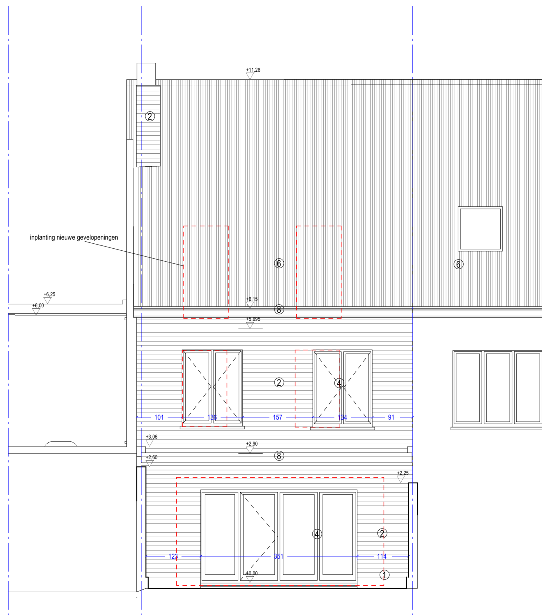
ACHTERGEVEL (tuinzijde) - bestaande toestand
