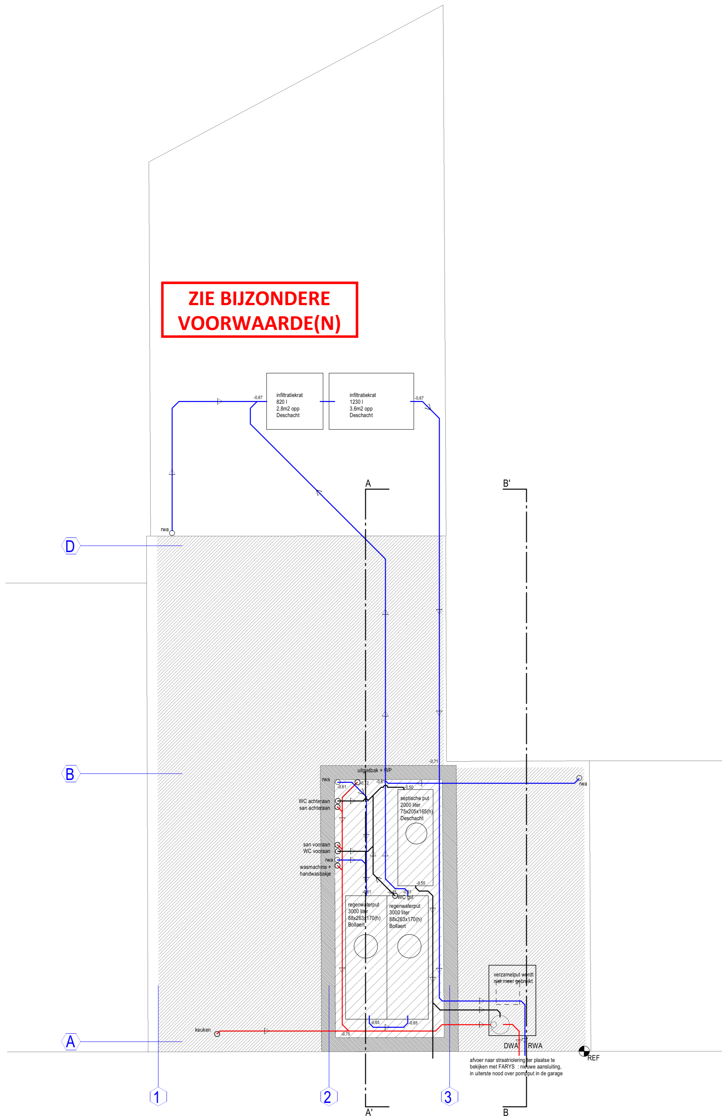
KELDER - nieuwe toestand
