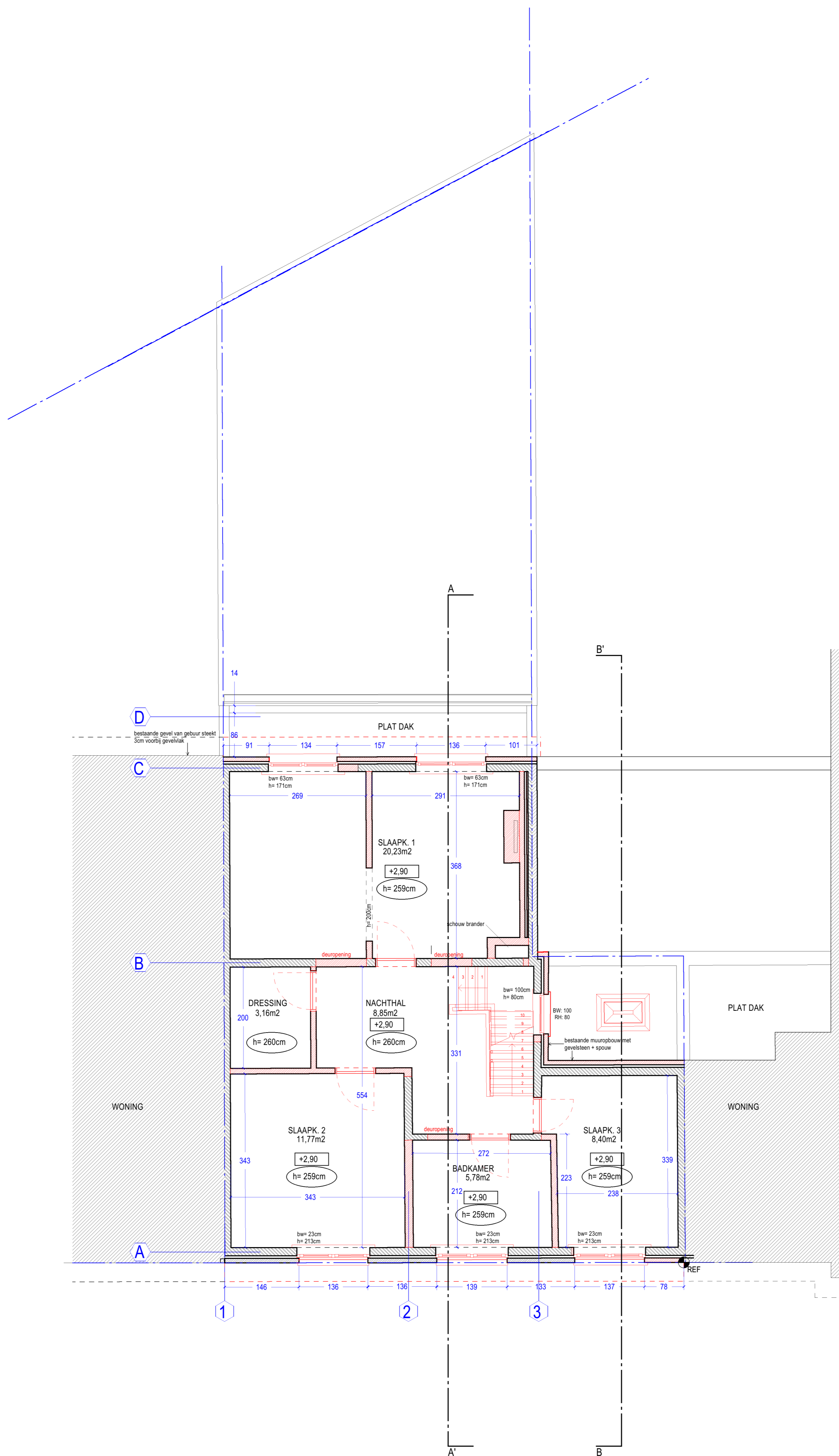
1ste VERDIEPING - bestaande toestand
