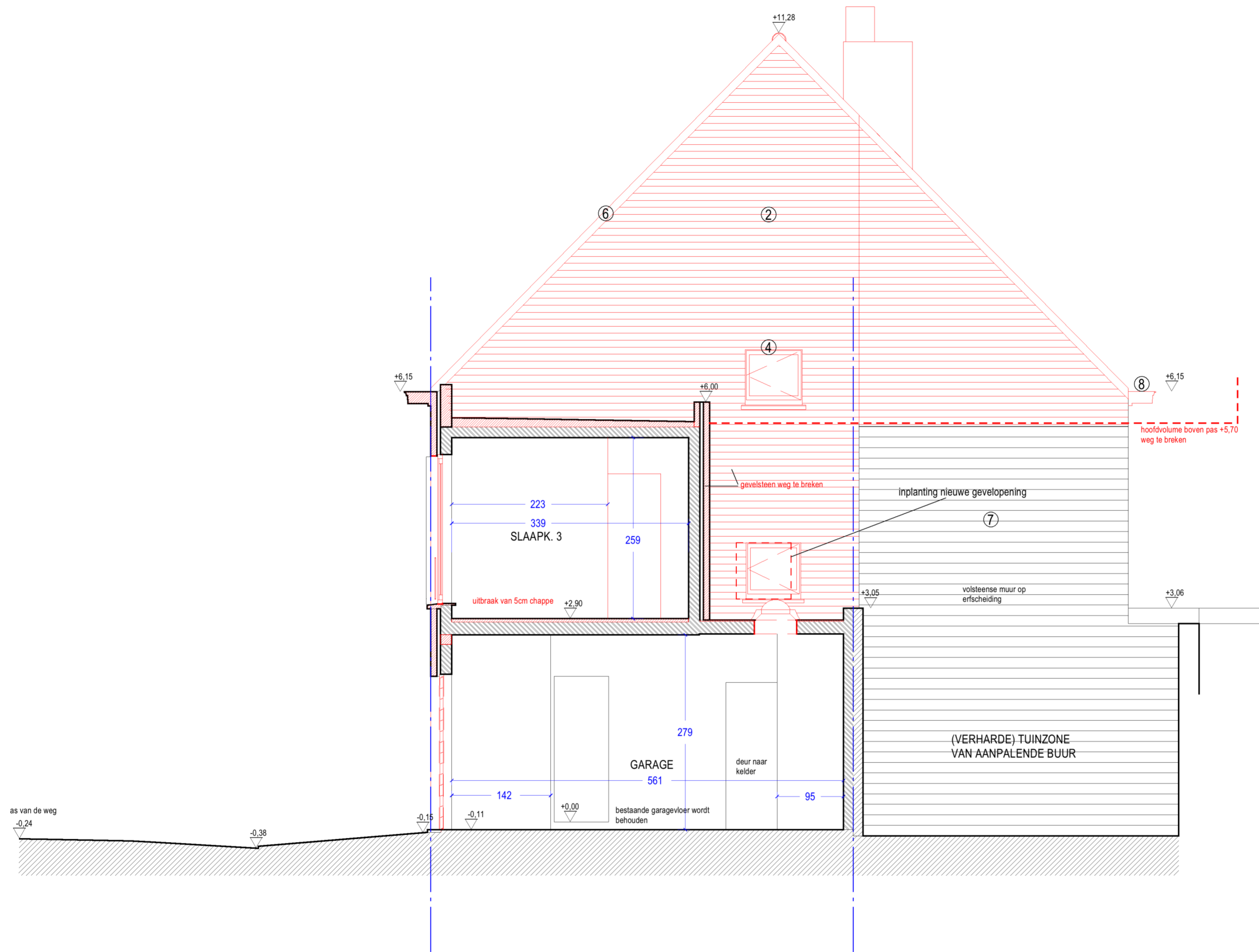
DOORSNEDE B-B' - bestaande toestand
