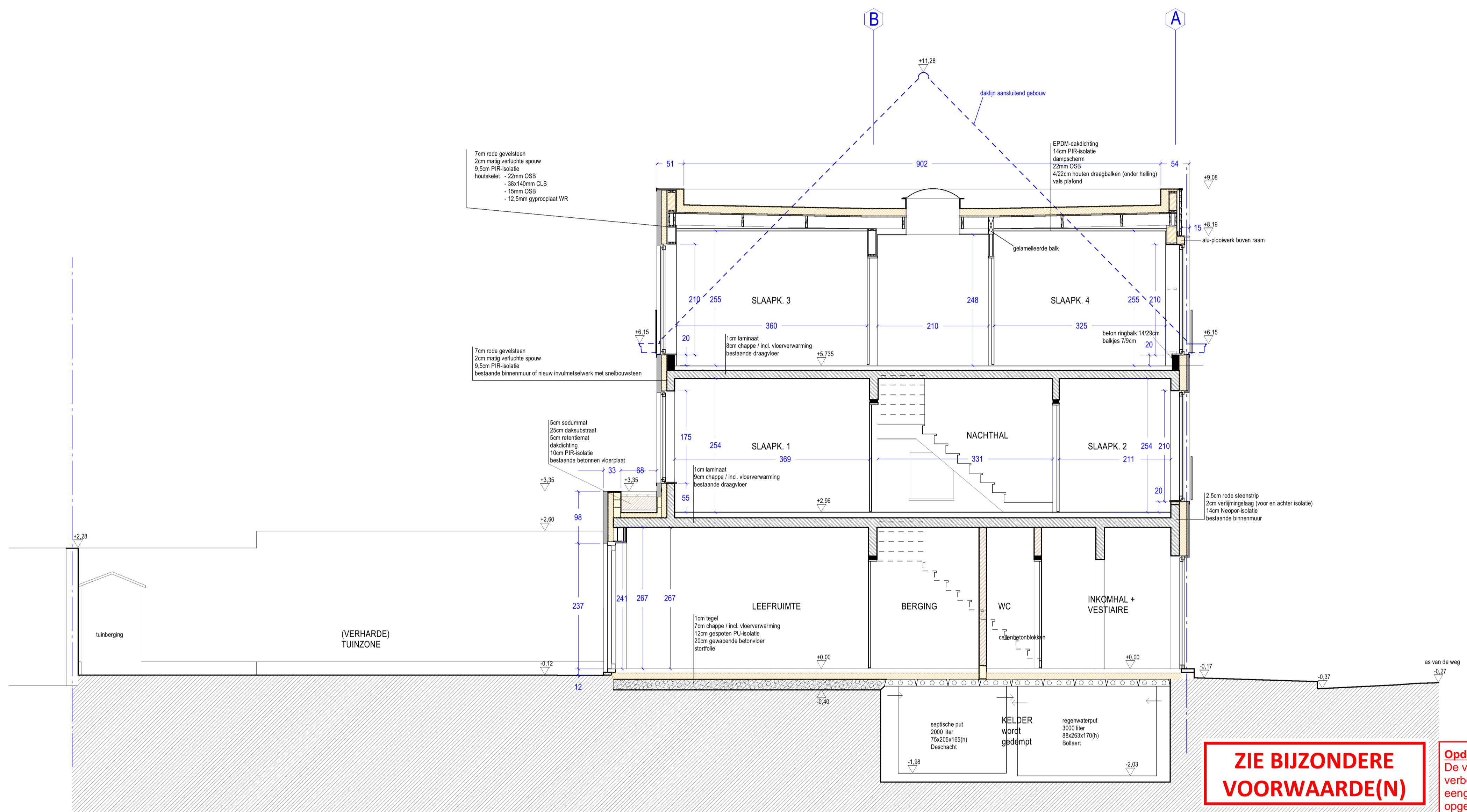
DOORSNEDE A-A' - bestaande toestand
