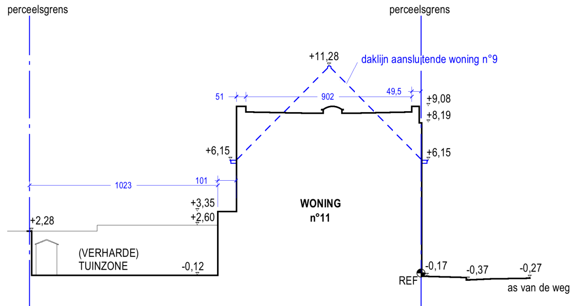
TERREINPROFIEL - nieuwe toestand
