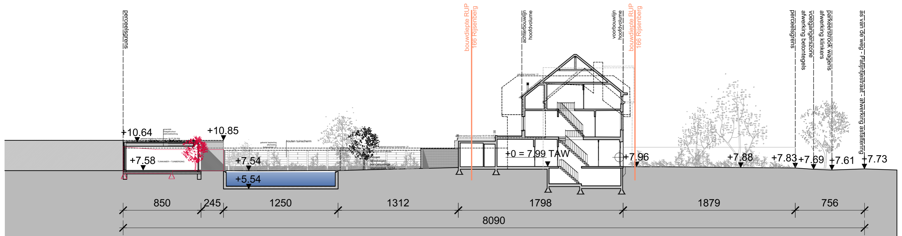
TERREINPROFIEL TP01 -nieuwe toestand (tuinkamer + zwembad)
