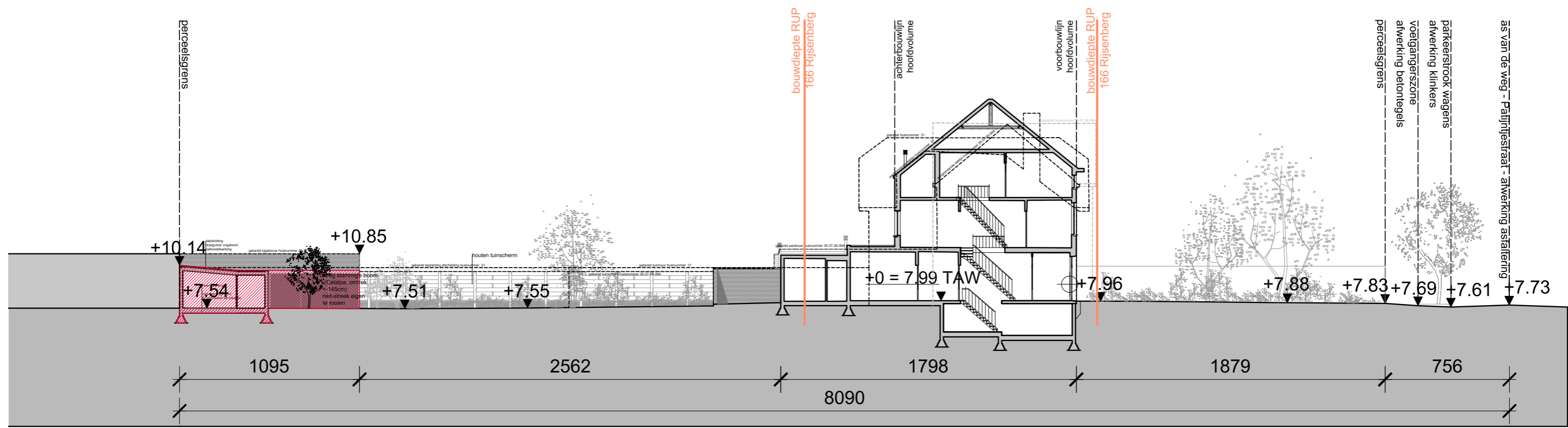
TERREINPROFIEL TP01 -bestaande toestand 0 2 10 te slopen
