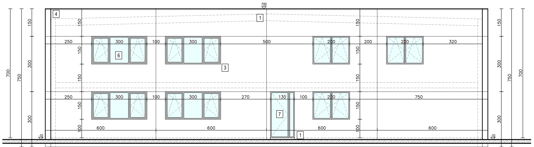
VOORGEVEL Vergunde toestand Schaal 1/100
