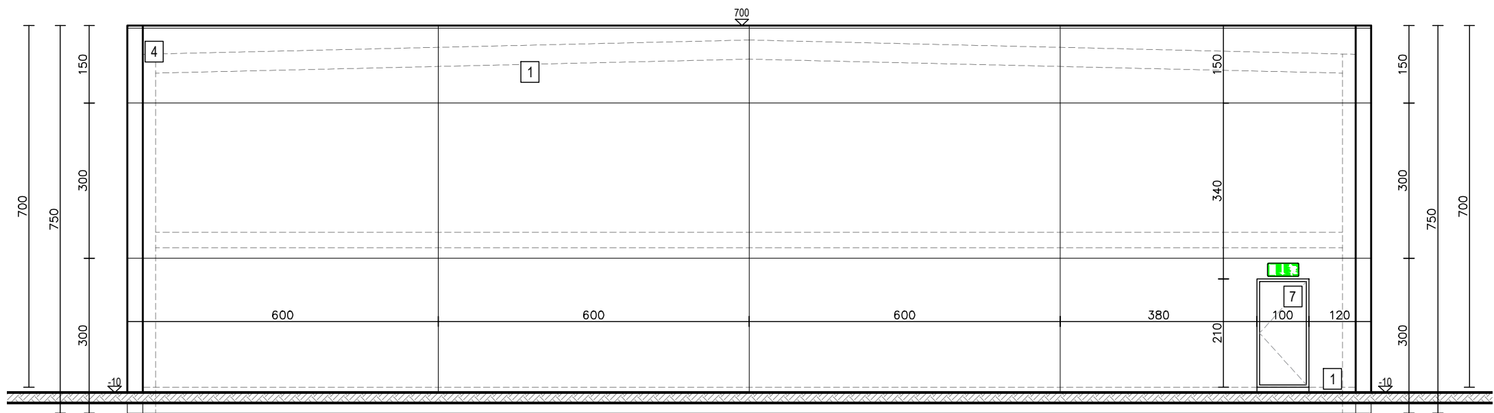
ACHTERGEVEL Vergunde toestand Schaal 1/100
