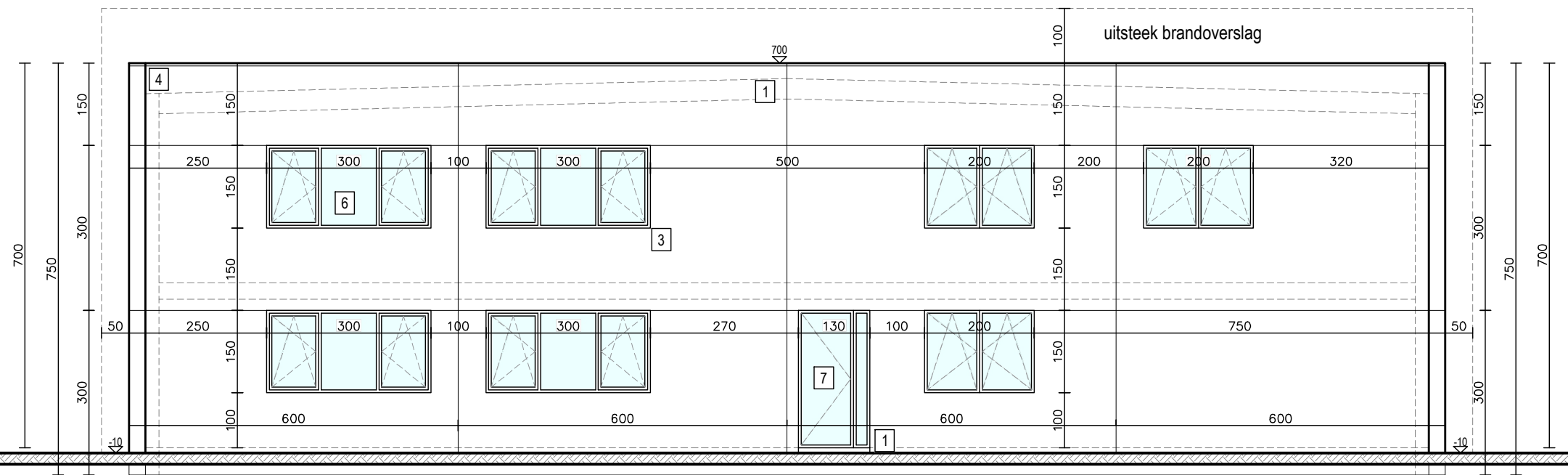
VOORGEVEL Nieuwe toestand Schaal 1/100
