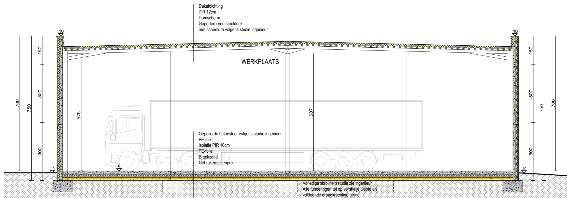
SNEDE AA Vergunde toestand Schaal 1/100
