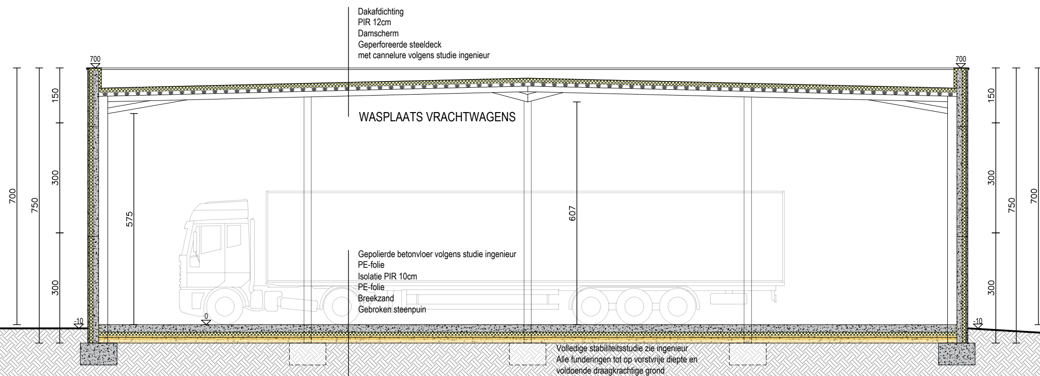
SNEDE AA Nieuwe toestand Schaal 1/100
