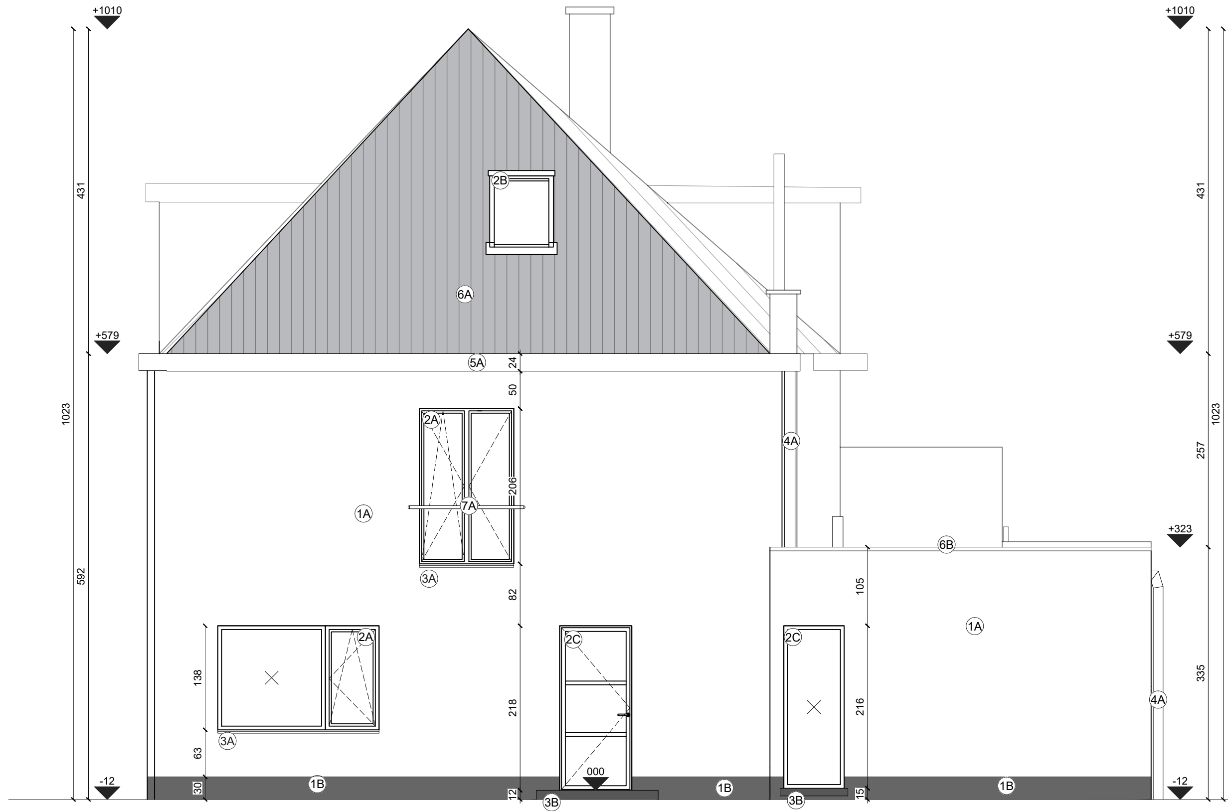
NIEUWE TOESTAND: GEVEL RECHTS schaal 1:50
