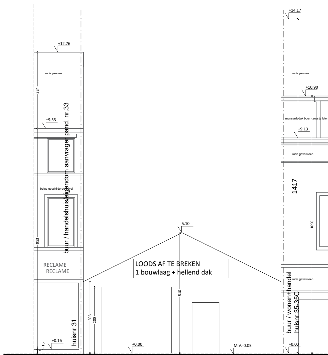
VOORGEVEL BESTAAND (loods)
