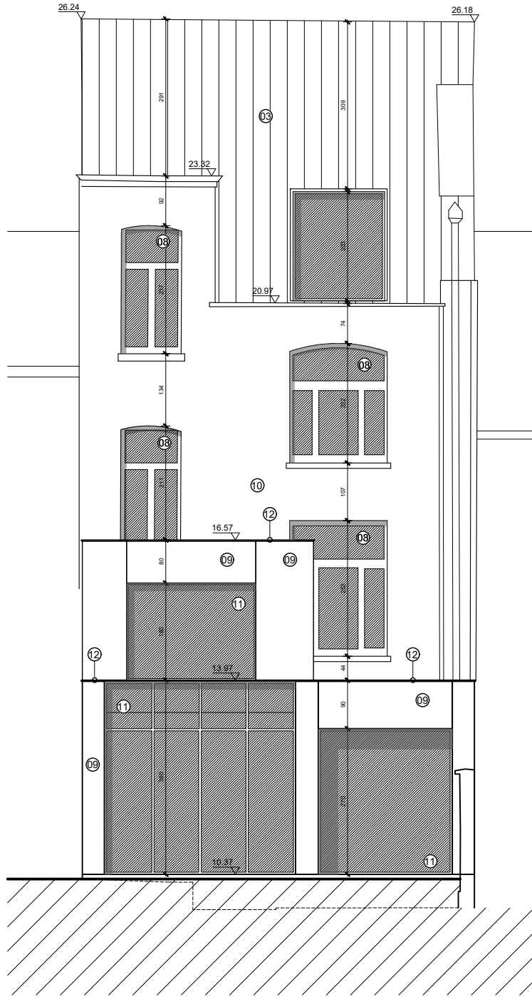
ZICHT ACHTERGEVEL NIEUWE TOESTAND
